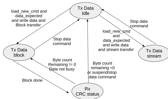
图 34.4-3. 数据发送状态机
