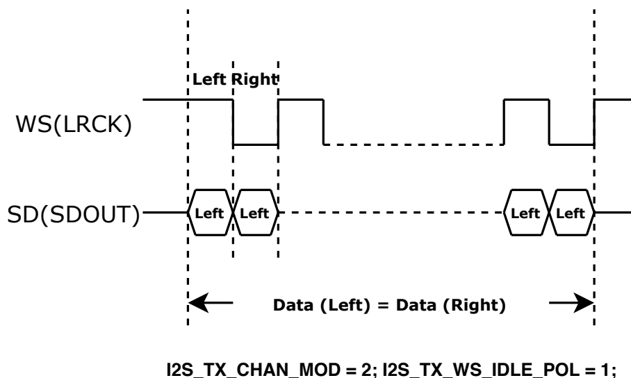
图 28.9-3. PDM 通道控制
