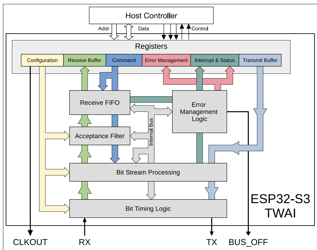
图 31.4-1. TWAI 概略图
