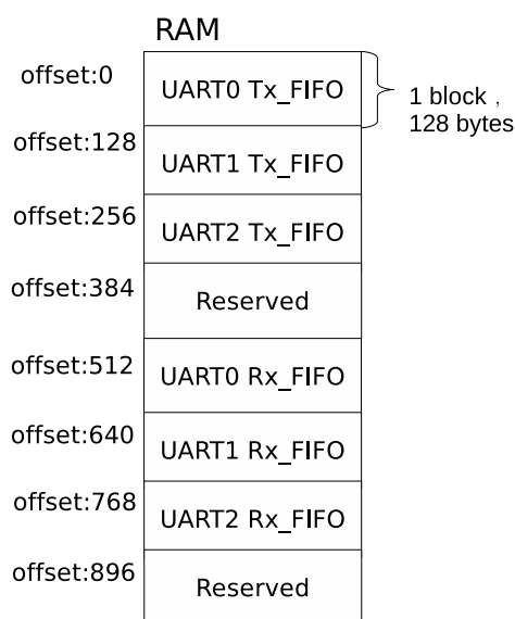
图 26.4-1. UART 共享 RAM 图
