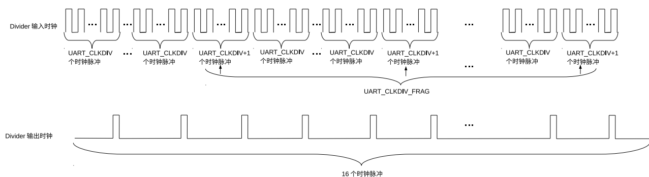
图 26.4-2. UART 控制器分频
