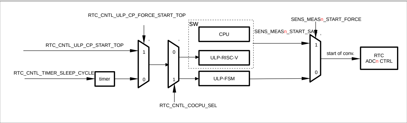
图 39.3-3. RTC SAR ADC 的功能概况
