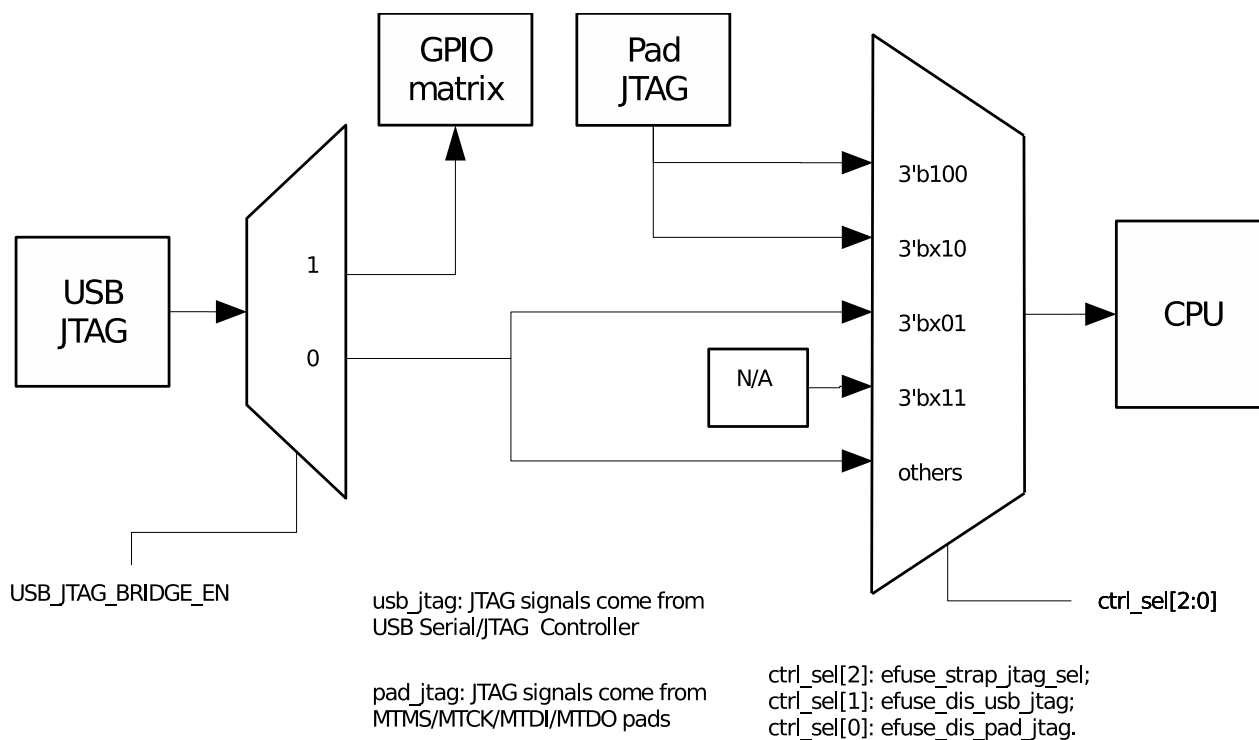
图 33.3-2. JTAG 信号传输
