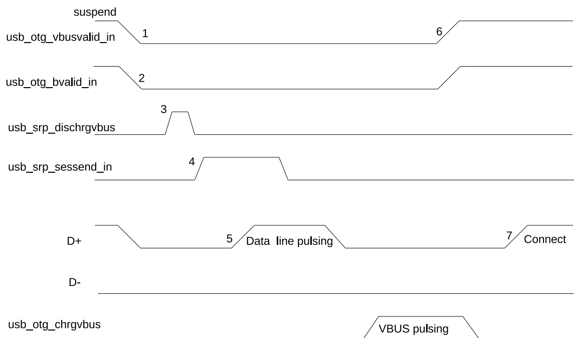
图 32.4-2. B 设备 SRP
