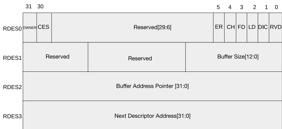
图 34.8-1. 链表结构
