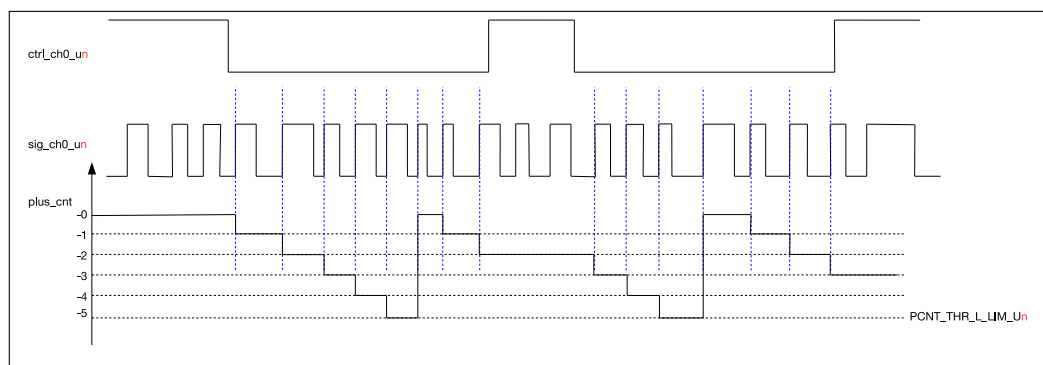
图 38.3-2. 通道 0 递减计数图
