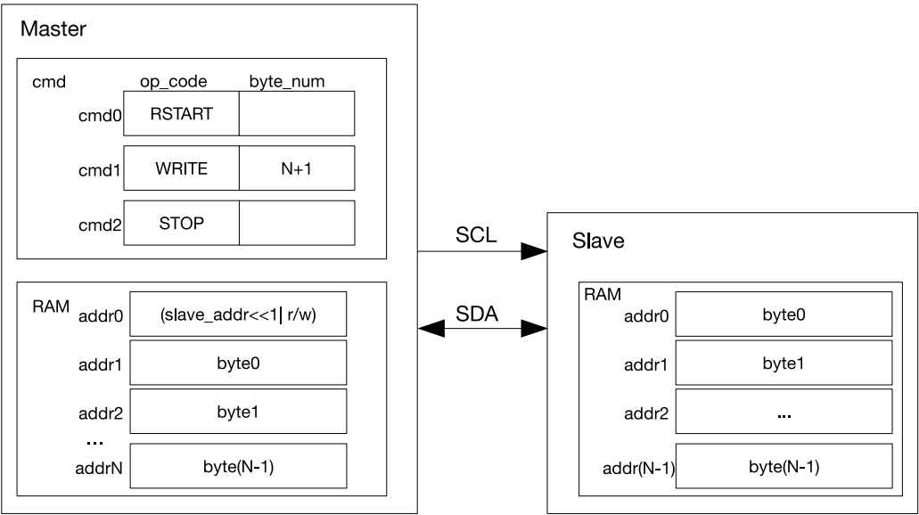
图 27.5-1. I2C 主机写 7 位寻址的从机
