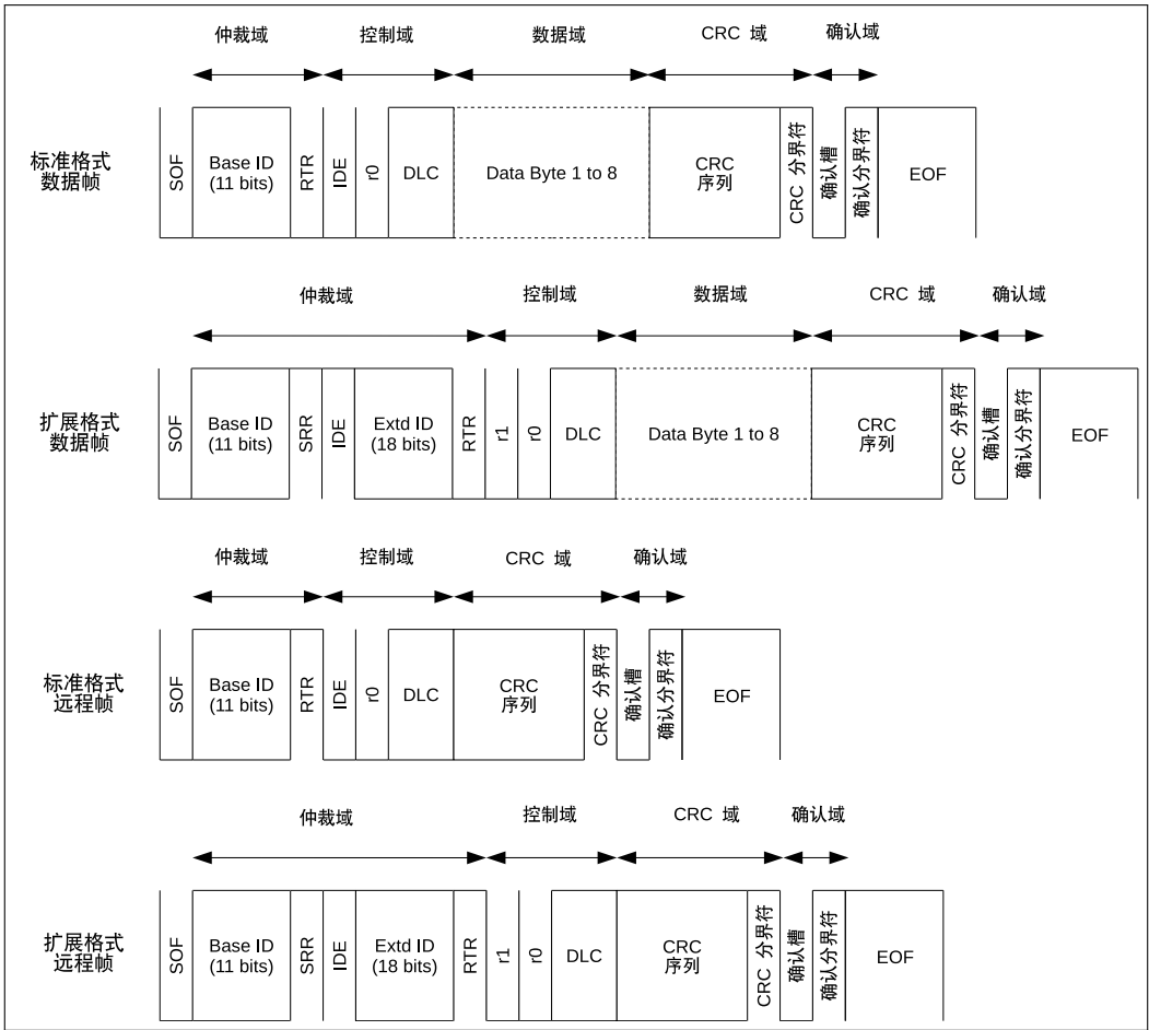
图 31.3-1. 数据帧和远程帧中的位域
