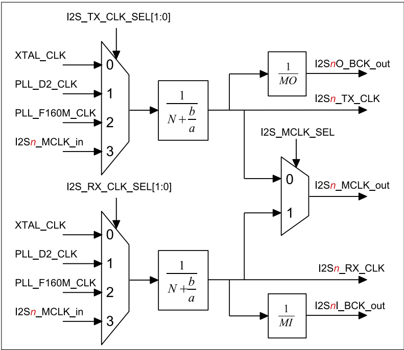
图 28.6-1. I2S n 时钟
