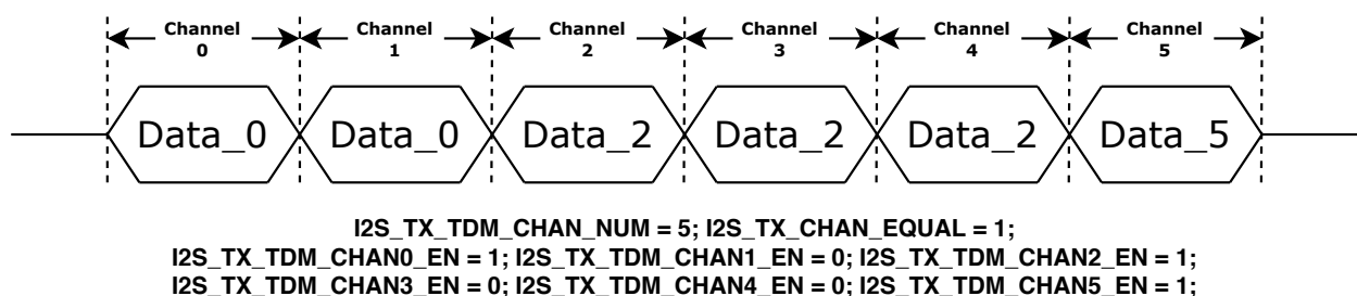
图 28.9-2. TDM 通道控制
