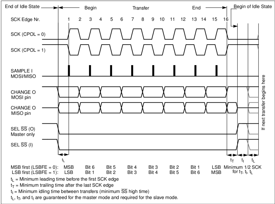
图 30.7-1. SPI 时钟模式 0 和时钟模式 2
