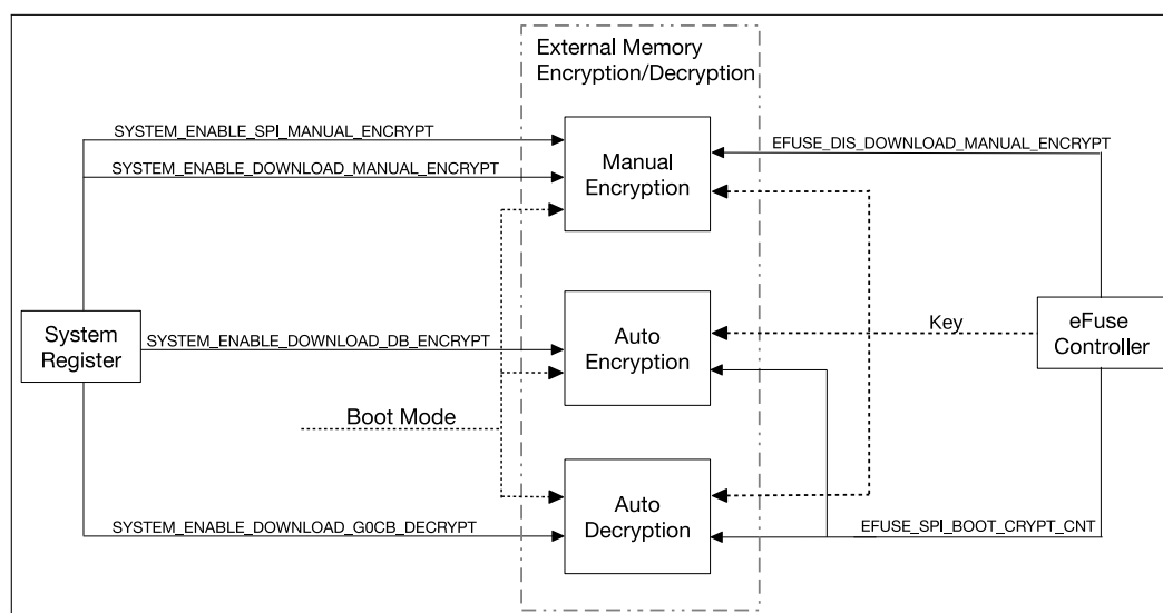
图 23.3-1. 片外存储器加解密工作配置
