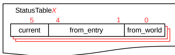
图 16.5-1. 世界切换记录表
