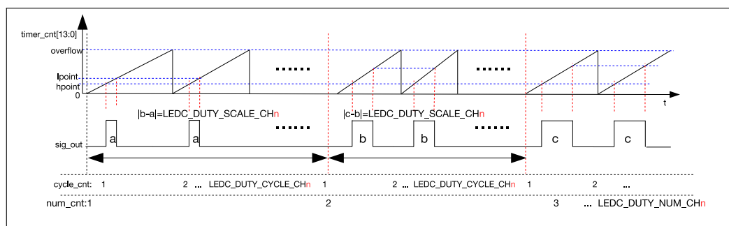
图 35.2-4. 输出信号占空比渐变图
