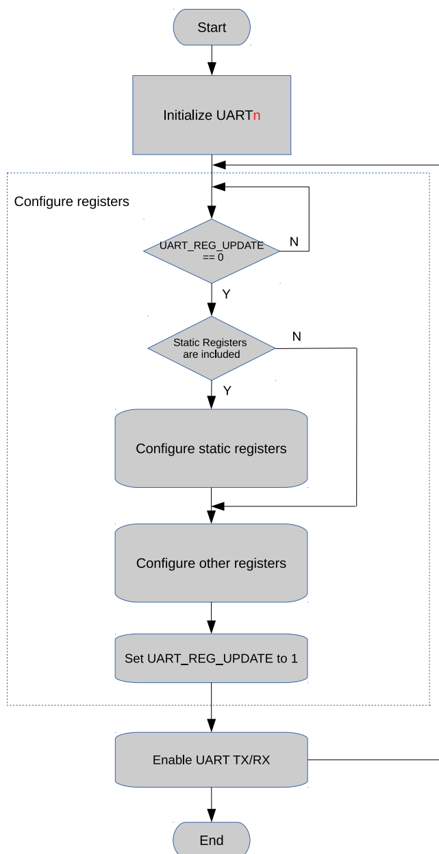
图 26.5-1. UART 编程流程
