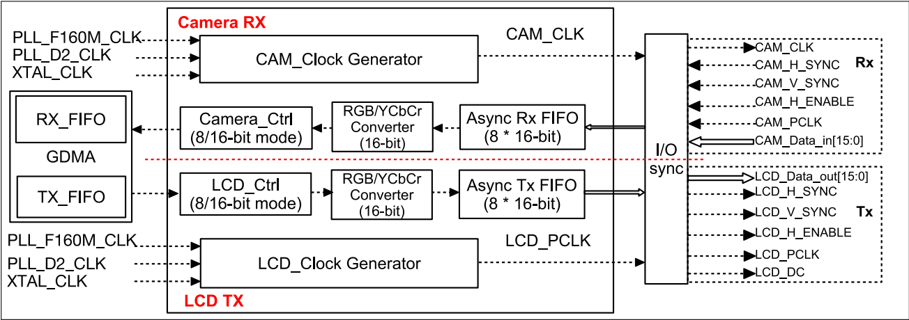
图 29.3-1. LCD_CAM 功能框图
