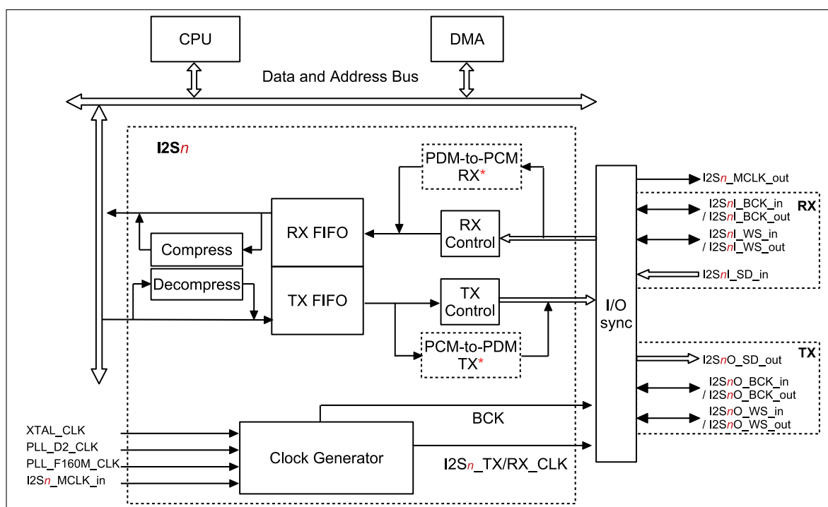
图 28.4-1. ESP32-S3 I2S 系统框图
