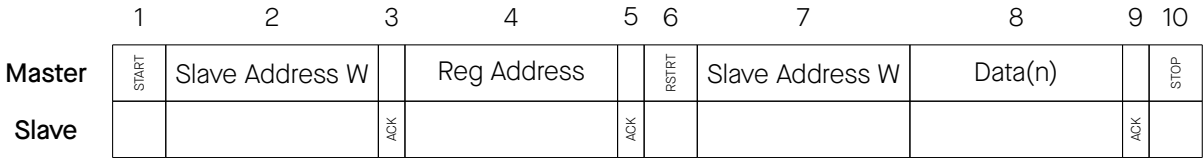
图 2.7-2. I2C 写操作
