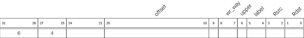
图 2.5-9. 指令类型 - 指定地址模式的数据存储
