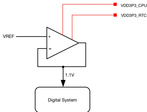
图 10.3-5. 数字调压器
