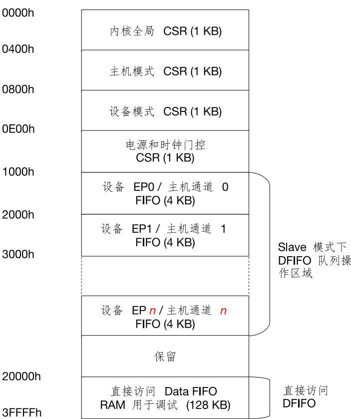
图 32.3-2. 内核地址映射
