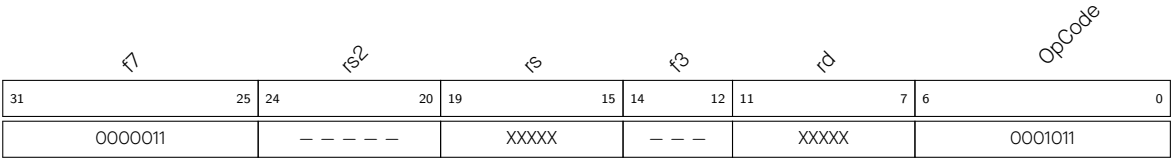
图 2.6-5. 中断指令 - Maskirq rd rs
