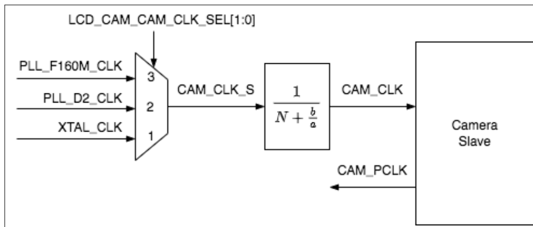
图 29.3-3. Camera 时钟
