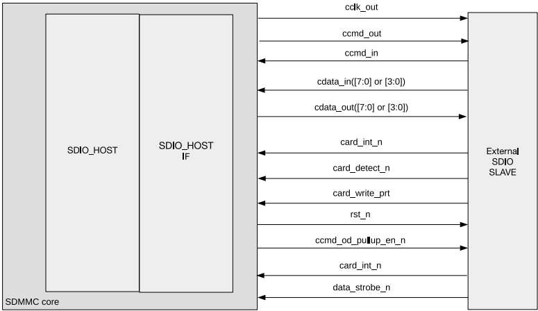
图 34.3-1. SD/MMC 控制器外部接口信号
