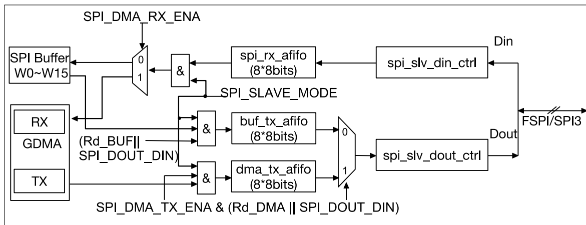
图 30.5-4. 从机模式下的数据流控制
