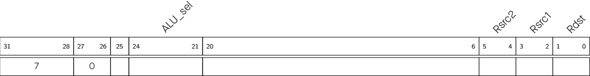
图 2.5-2. 指令类型 - 对寄存器数值的 ALU 运算
