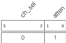
图 39.3-10. SAR ADC1 cmd1 配置示例
