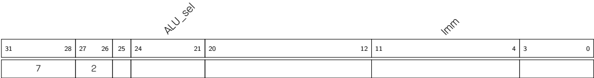
图 2.5-4. 指令类型 - 对阶段计数器寄存器的 ALU 运算
