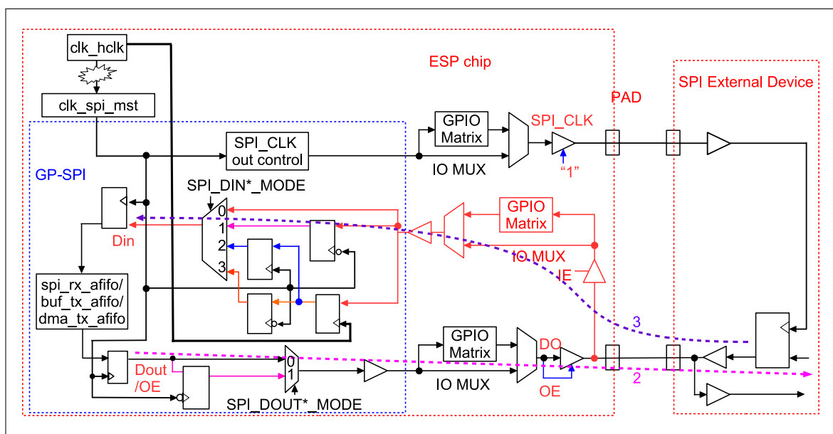
图 30.8-1. GP-SPI 主机模式下时序补偿控制图
