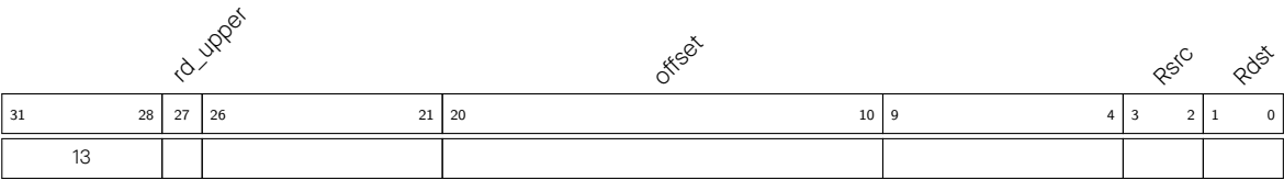
图 2.5-10. 指令类型 - LD
