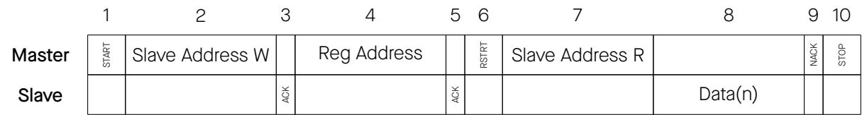
图 2.7-1. I2C 读操作
