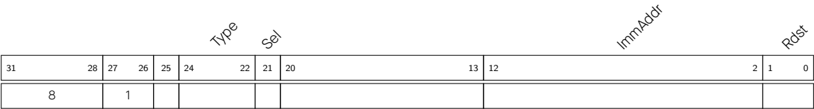
图 2.5-11. 指令类型 - JUMP
