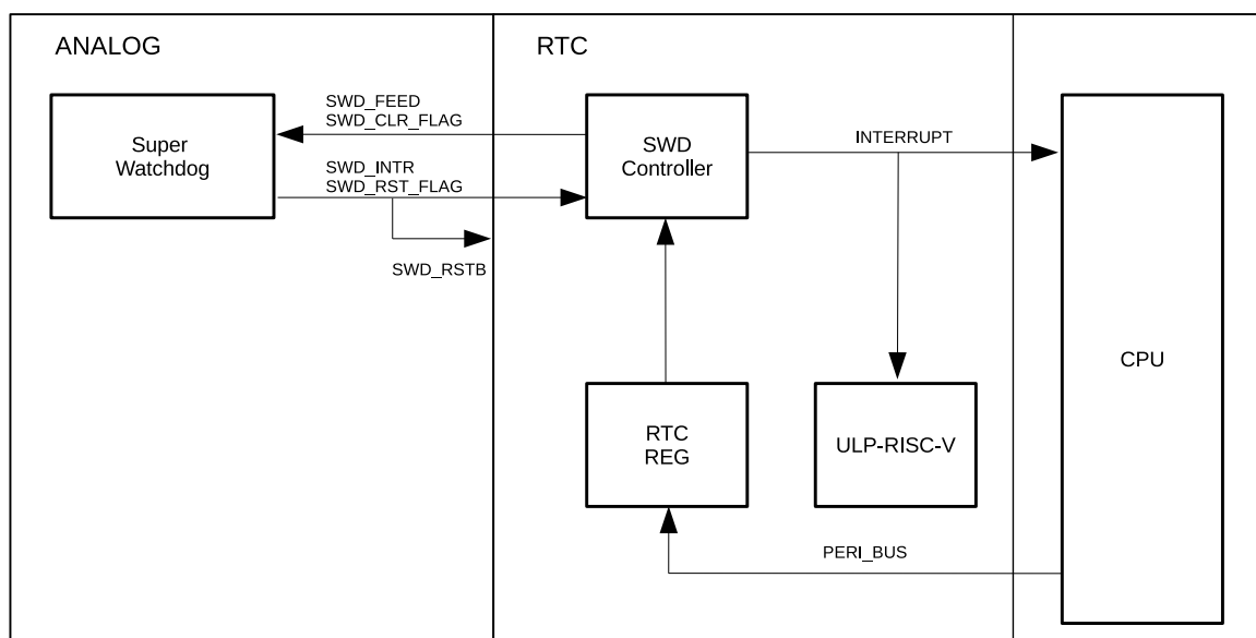
图 13.3-1. SWD 控制器结构
