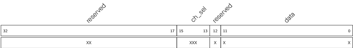
图 39.3-11. DMA 数据格式
