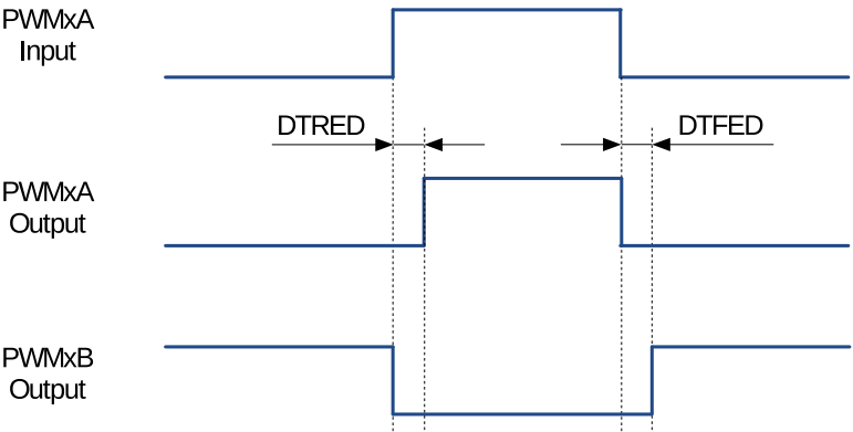
图 36.3-22. 高电平有效互补 (AHC) 死区波形
