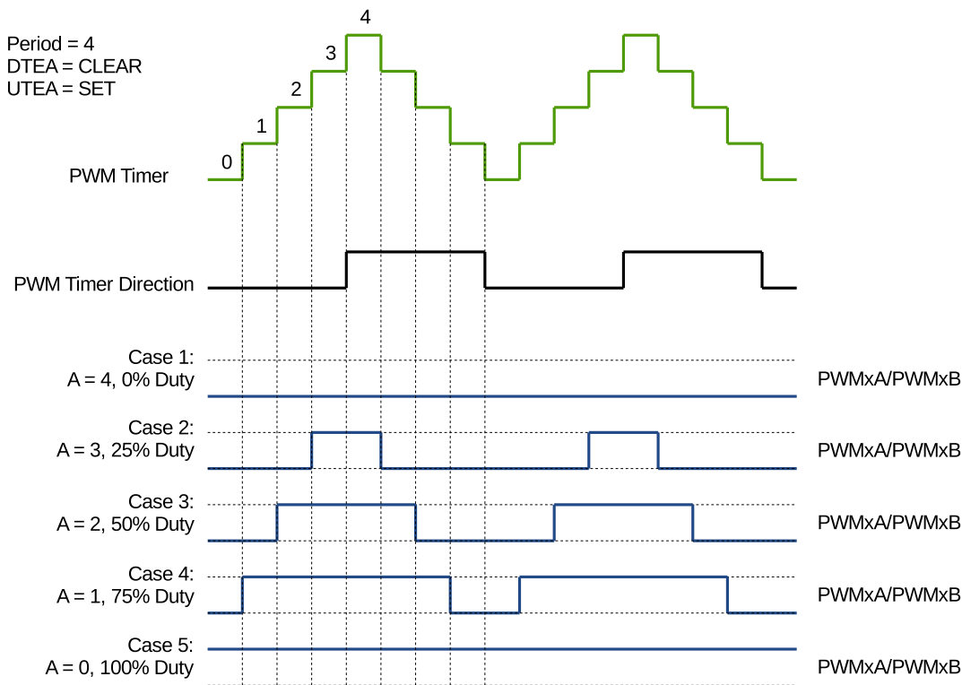
图 36.3-14. 递增递减模式下的对称波形
