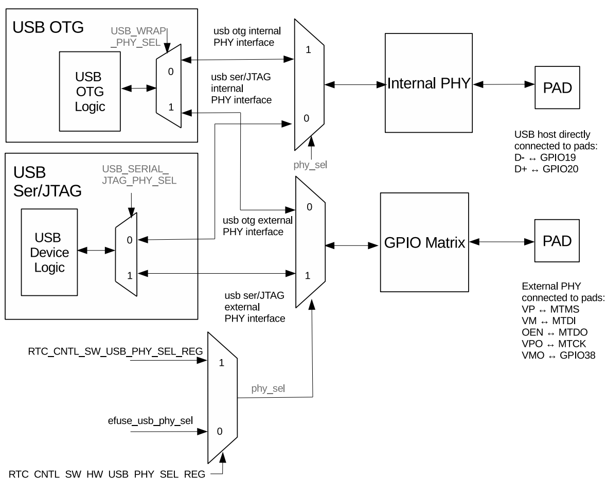
图 33.3-1. USB 串口/JTAG 与 USB-OTG 内部/外部 PHY 连接图
