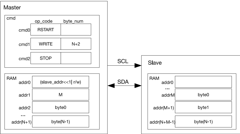
图 27.5-3. I2C 主机写 7 位双地址寻址从机
