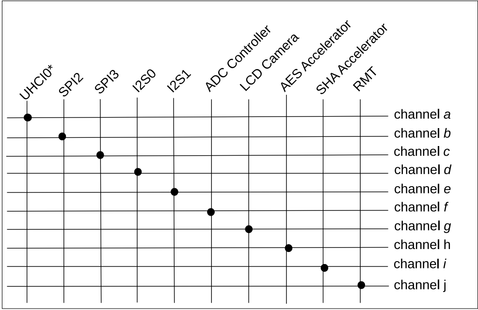
图 4.3-2. 具有 GDMA 功能的外设
