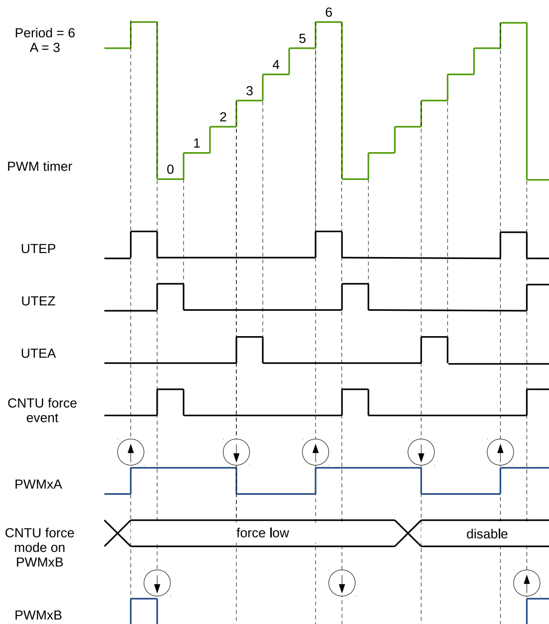
图 36.3-20. CNTU 在 PWMxB 输出上软件强制事件示例
