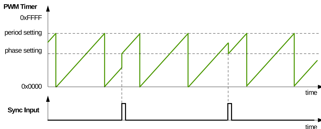
图 36.3-6. 递增计数模式波形
