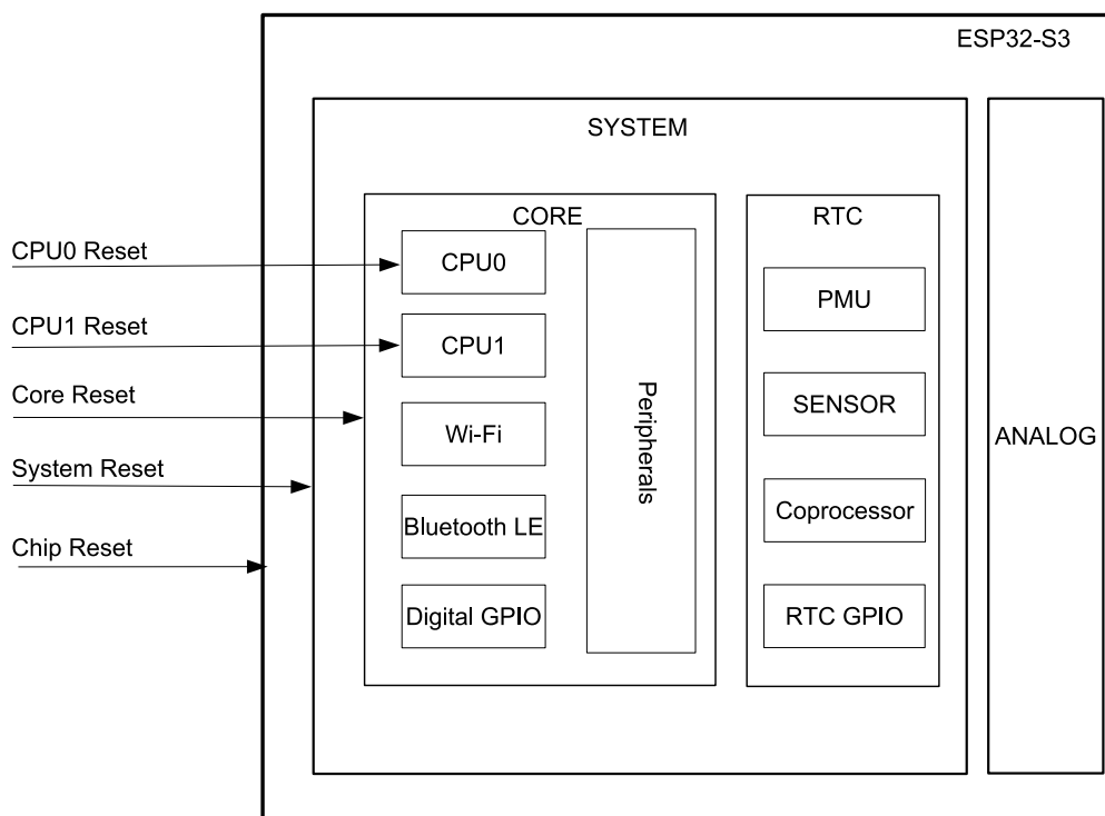
图 7.1-1. 四种复位等级
