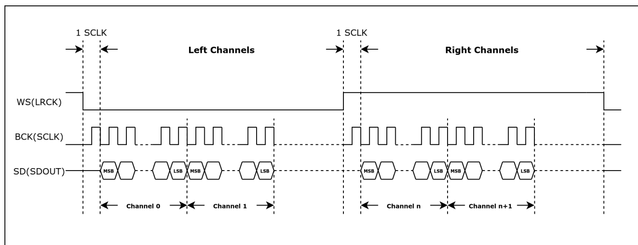
图 28.5-1. 时序图 – TDM Philips 标准
