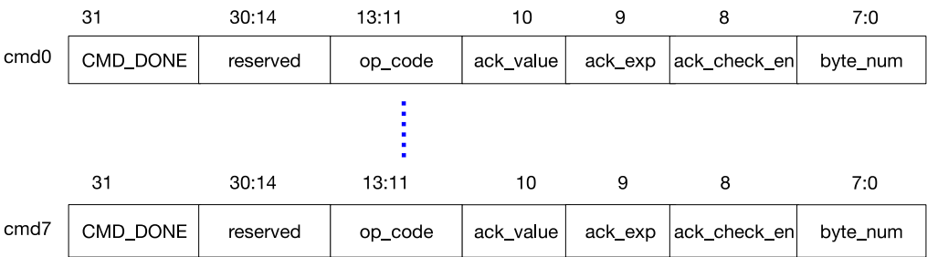
图 27.4-2. I2C 命令寄存器结构
