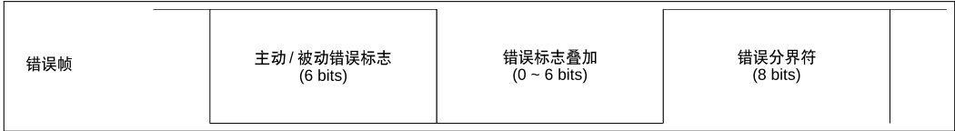
图 31.3-2. 错误帧中的位域
