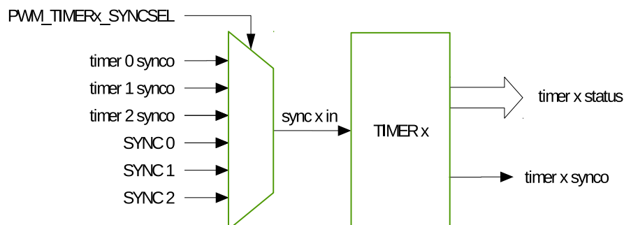
图 36.3-2. 定时器模块
