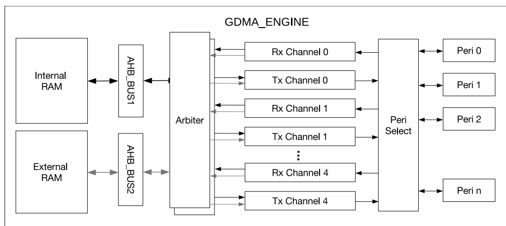
图 3.3-1. GDMA 引擎的架构
