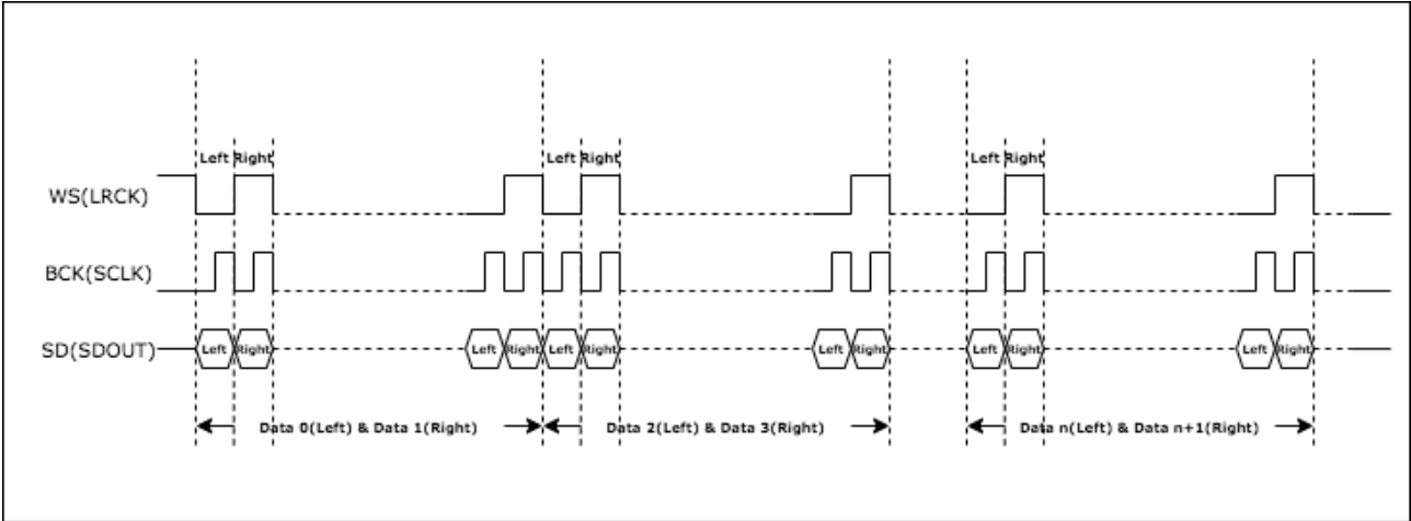
图 28.5-4. 时序图 – PDM 标准
