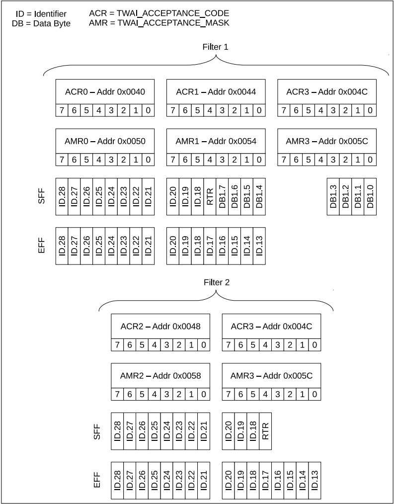
图 31.5-3. 双滤波模式
