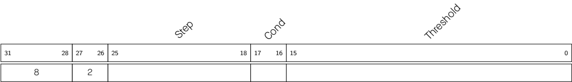
图 2.5-13. 指令类型 - JUMPS
