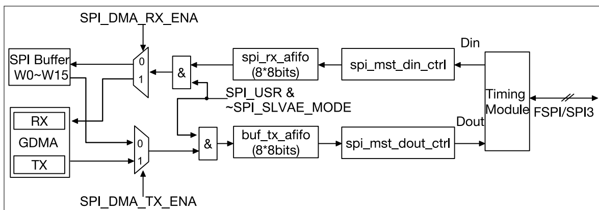
图 30.5-3. 主机模式下的数据流控制
