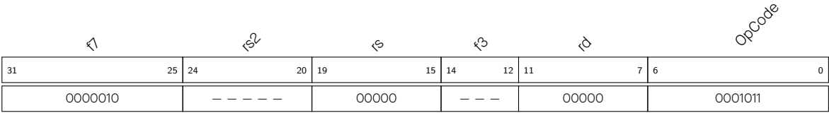
图 2.6-4. 中断指令 - retirq
