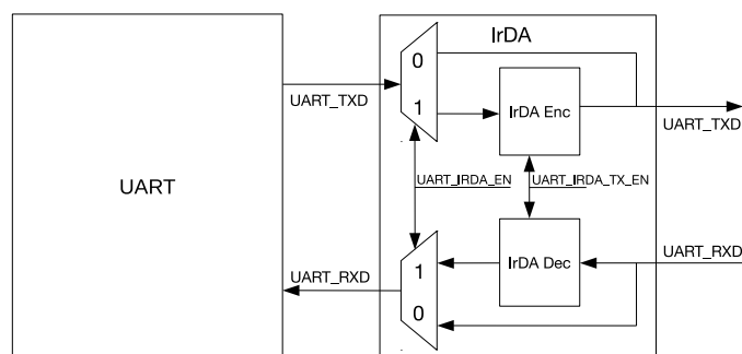
图 26.4-8. IrDA 编解码结构图
