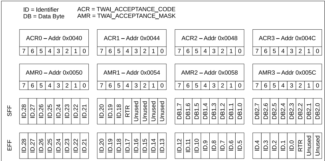
图 31.5-2. 单滤波模式
