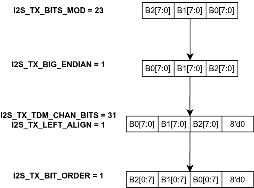
图 28.9-1. TX 数据格式控制
