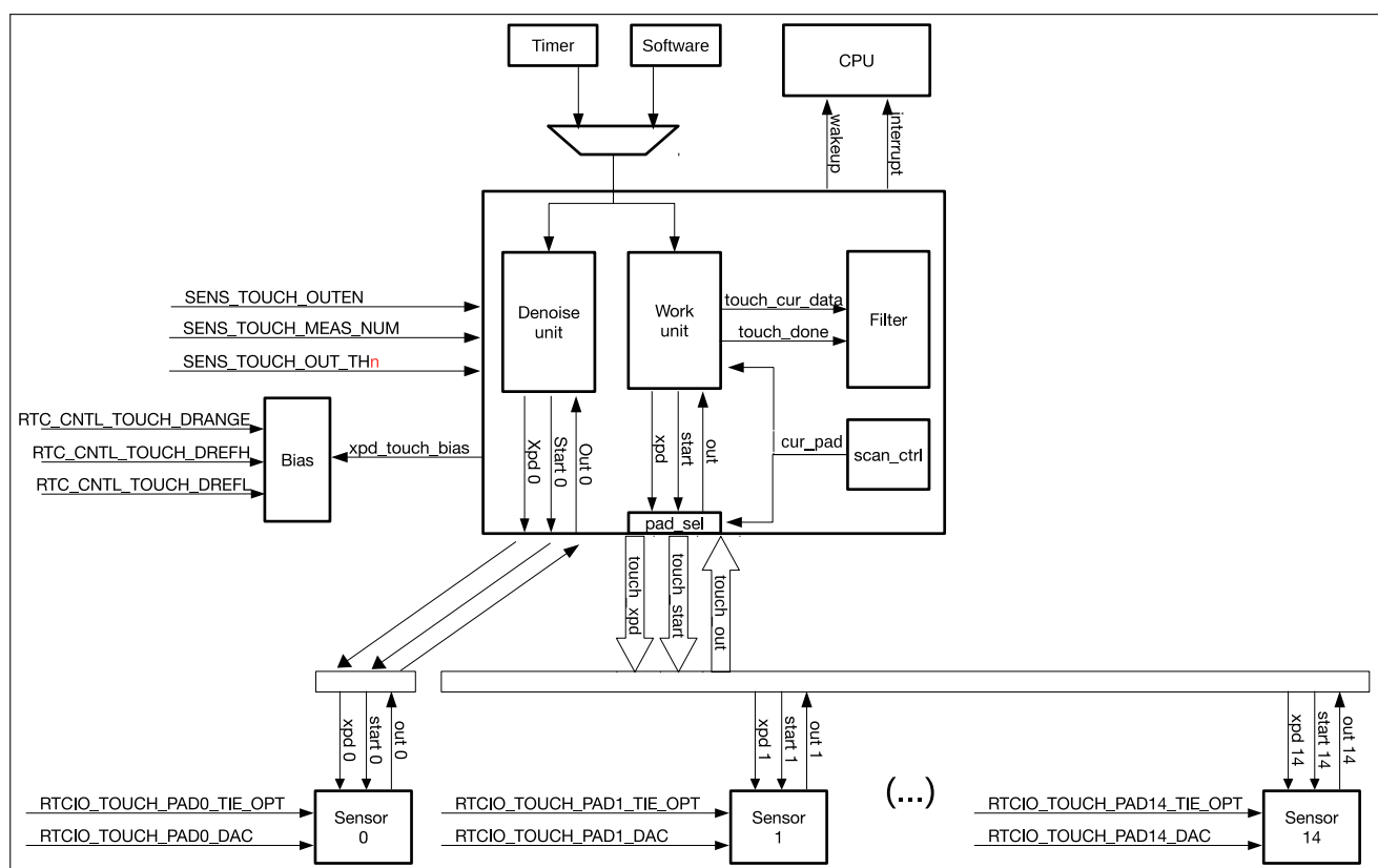
图 39.2-4. Touch FSM 的内部结构
