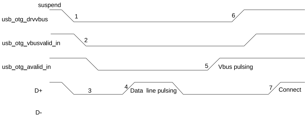
图 32.4-1. A 设备 SRP
