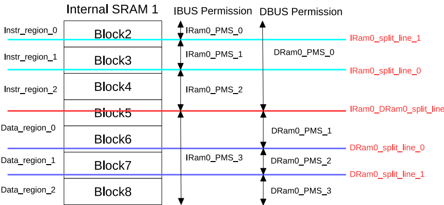
图 15.3-1. Internal SRAM1 的区域分割示意图
