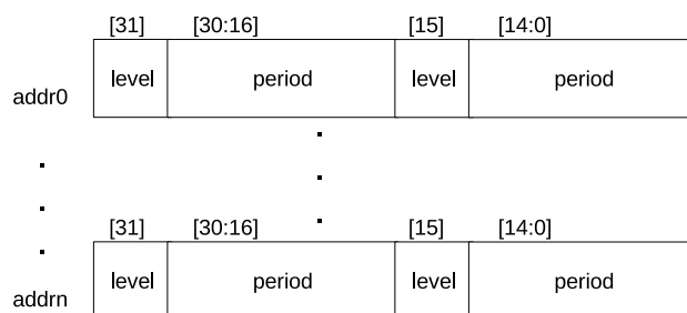
图 37.3-2. RAM 中脉冲编码结构
