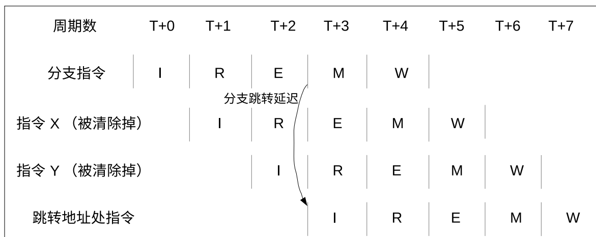
图 1.7-3. 控制冒险
