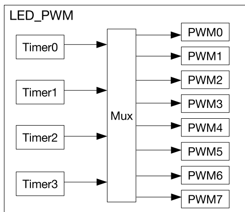
图 35.1-1. LED PWM 控制器架构
