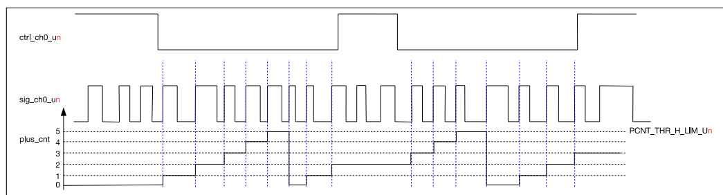
图 38.3-1. 通道 0 递增计数图
