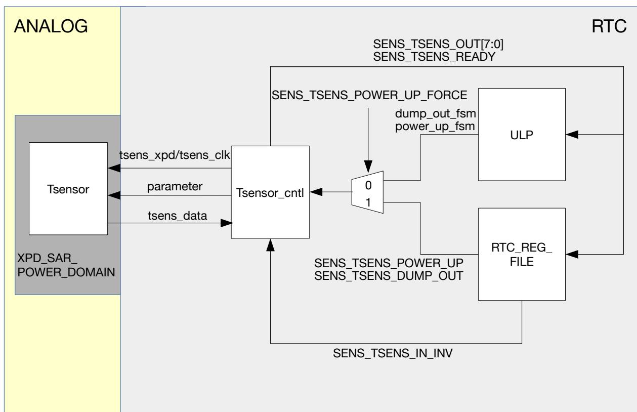
图 39.4-1. 温度传感器结构
