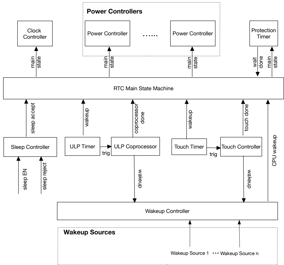
图 10.3-2. 电源管理单元的主要工作流程
