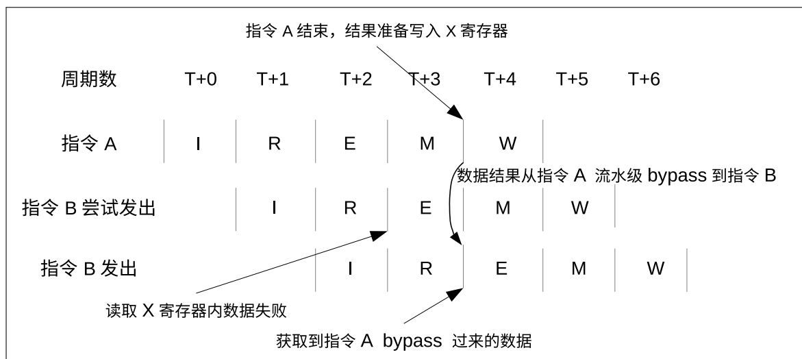
图 1.7-1. 指令操作数依赖导致内部锁
