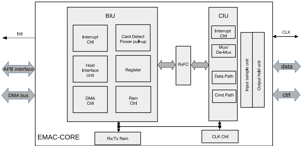
图 34.4-1. SDIO 主机结构框图
