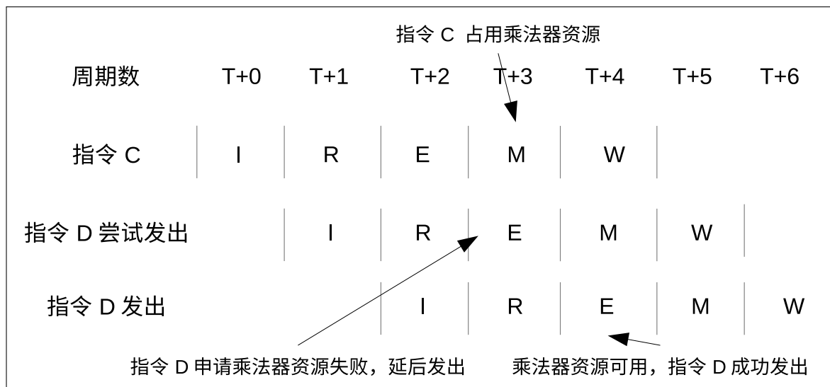
图 1.7-2. 硬件资源冒险
