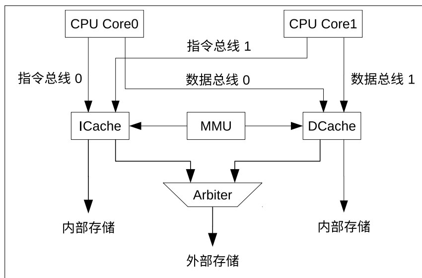
图 4.3-1. Cache 系统框图
