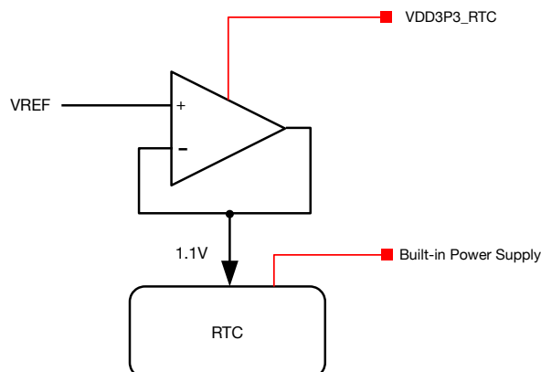
图 10.3-6. 低功耗调压器
