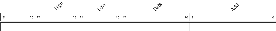
图 2.5-20. 指令类型 - REG_WR
