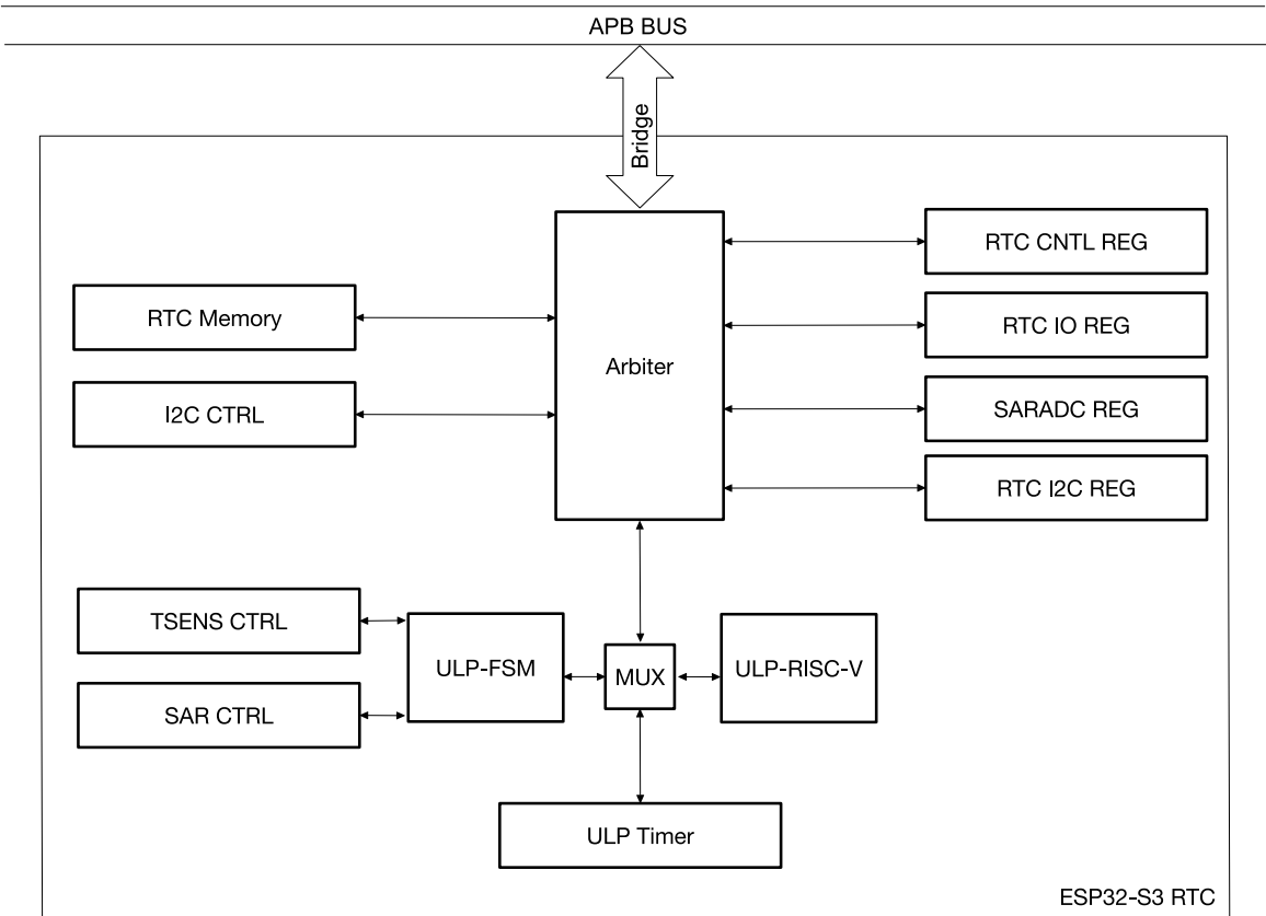
图 2.2-1. 超低功耗协处理器基本架构
