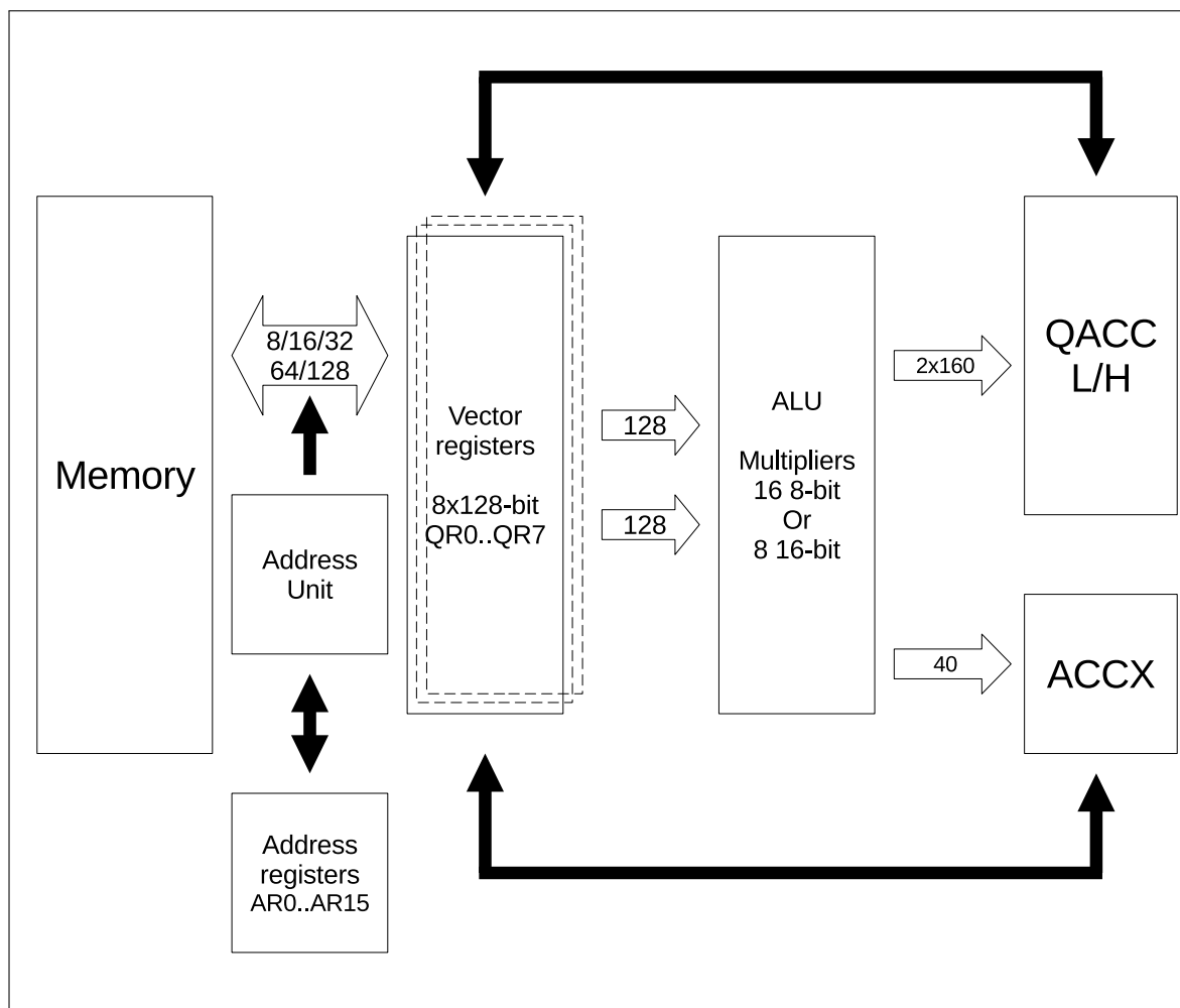
图 1.3-1. PIE 内部描述 (MAC)
