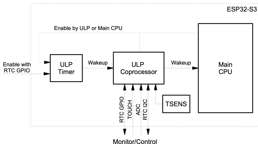
图 2.1-1. 超低功耗协处理器概图
