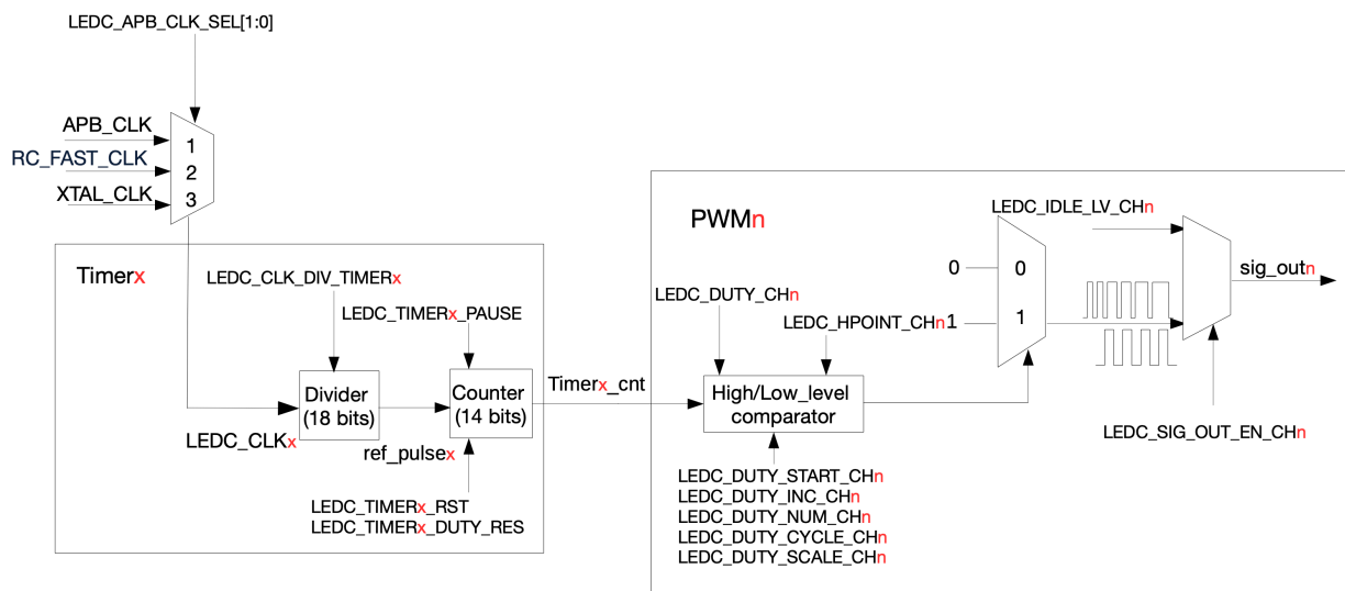
图 35.2-1. 定时器和 PWM 生成器功能块
