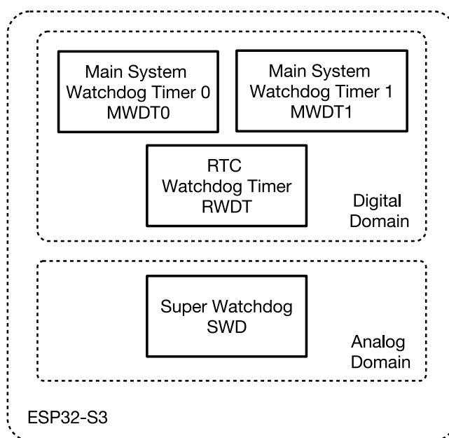
图 13.1-1. 看门狗定时器概览
