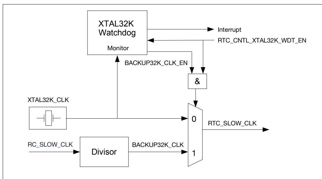
图 14.0-1. XTAL32K 看门狗定时器
