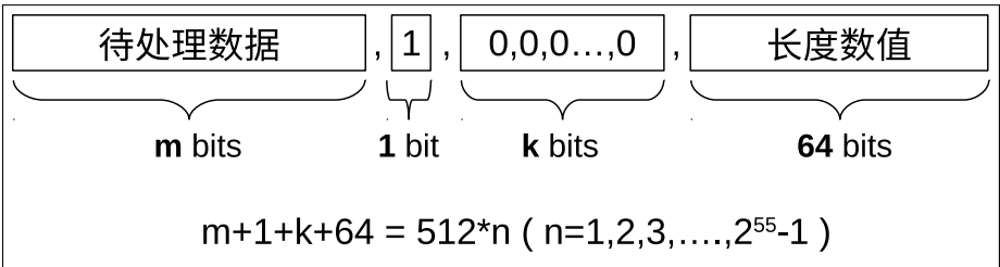
图 21.3-1. HMAC 附加填充比特示意图
