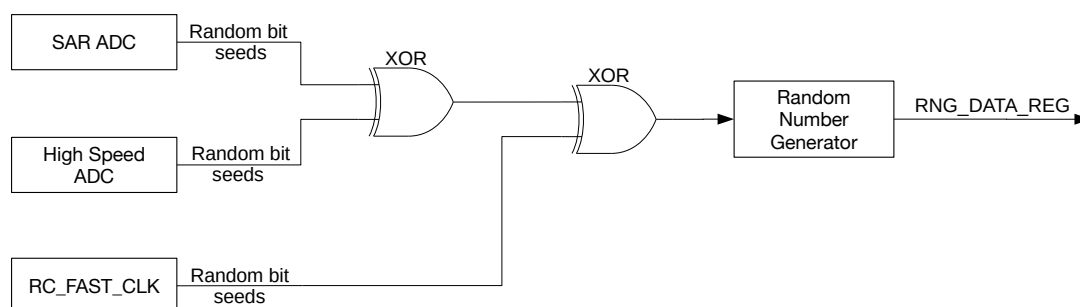
图 25.3-1. 噪声源
