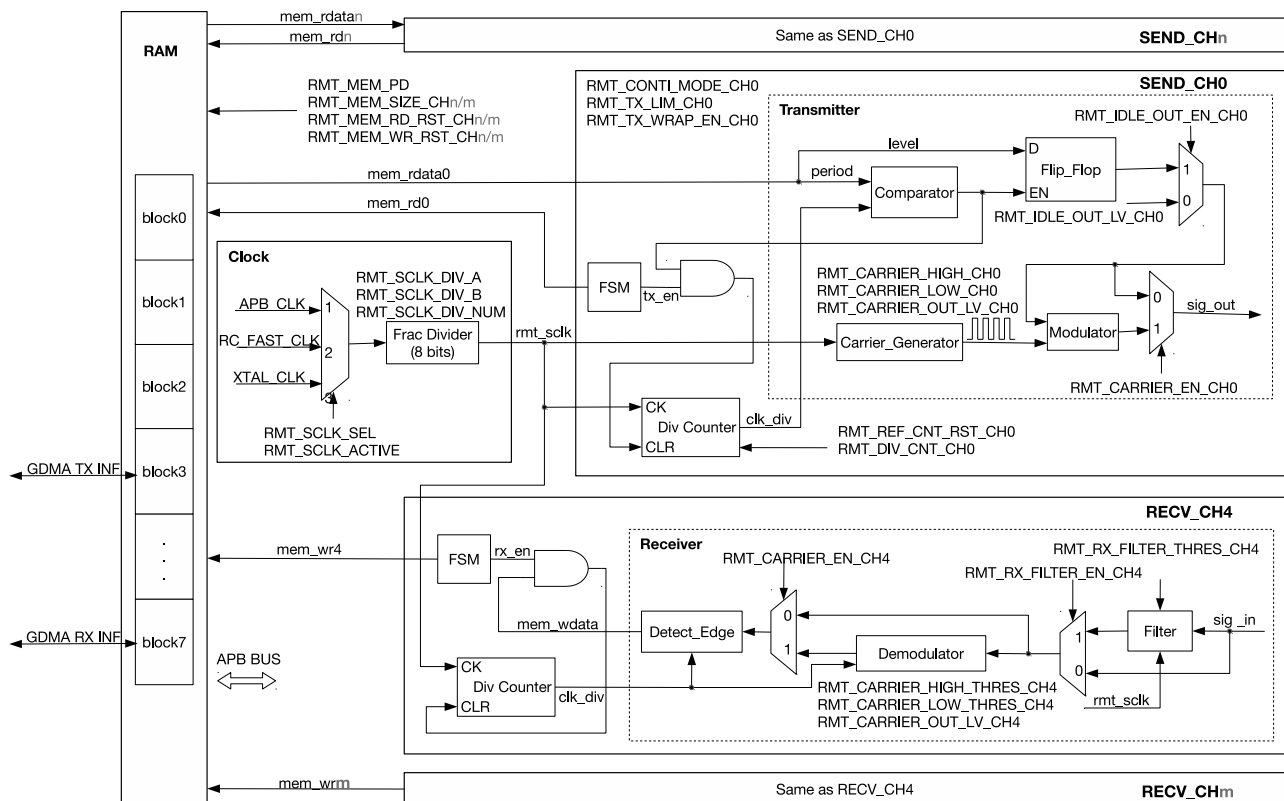
图 37.3-1. RMT 结构框图
