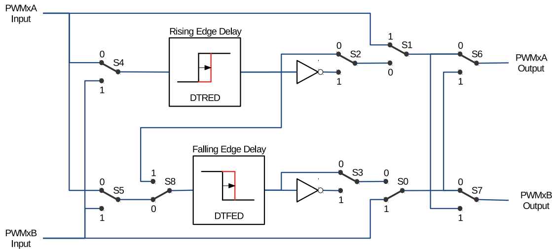
图 36.3-21. 死区模块的开关拓扑
