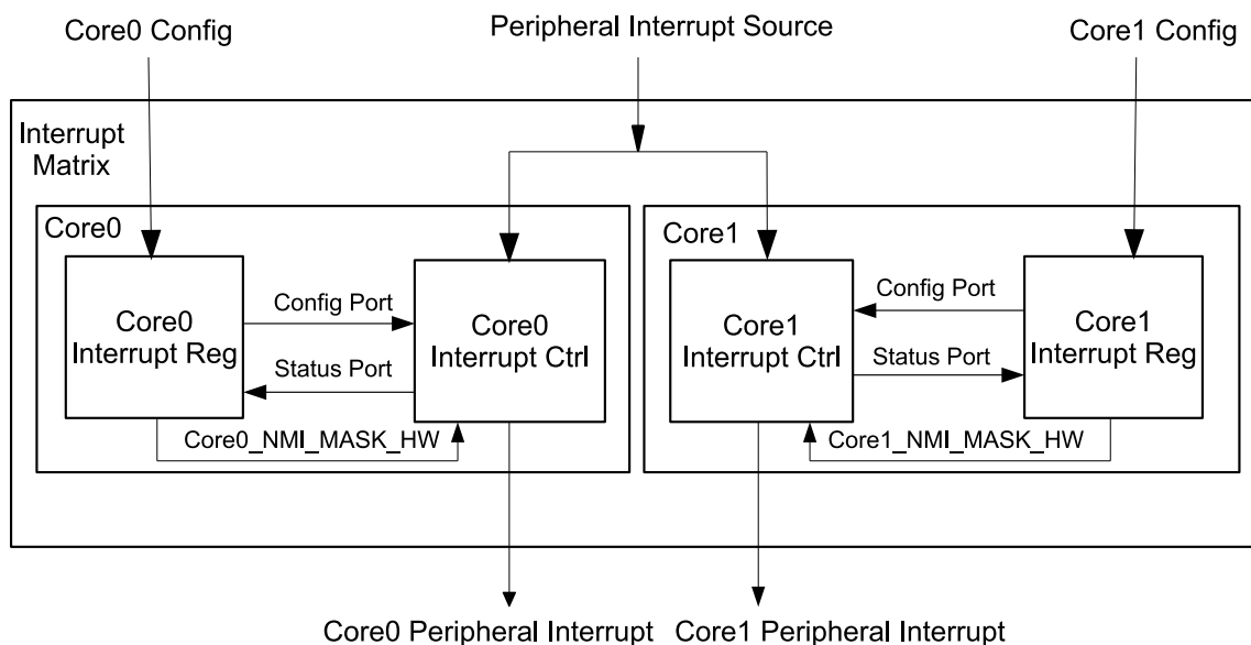
图 9.2-1. 中断矩阵结构图
