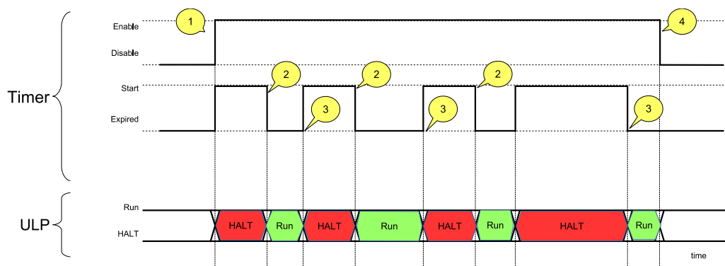
图 2.4-1. 协处理器睡眠和唤醒流程
