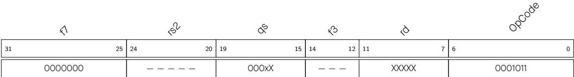
图 2.6-2. 中断指令 - getq rd, qs
