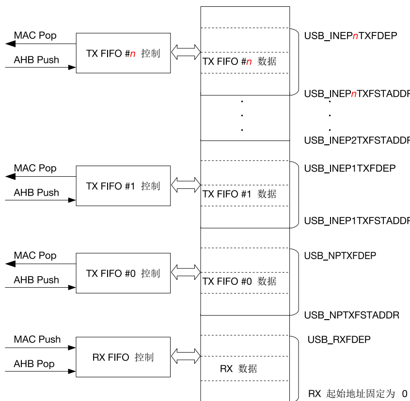
图 32.3-4. 设备模式 FIFO
