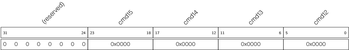
图 39.3-7. APB_SARADC_SAR1_PATT_TAB4_REG 与样式 12 - 15
