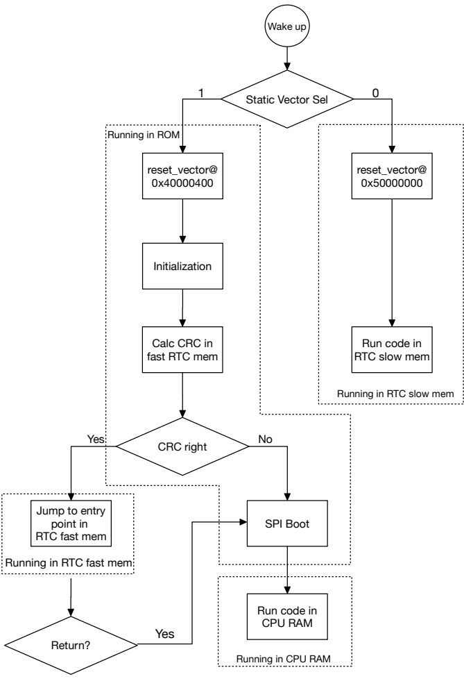
图 10.6-1. ESP32-S3 启动流程图
