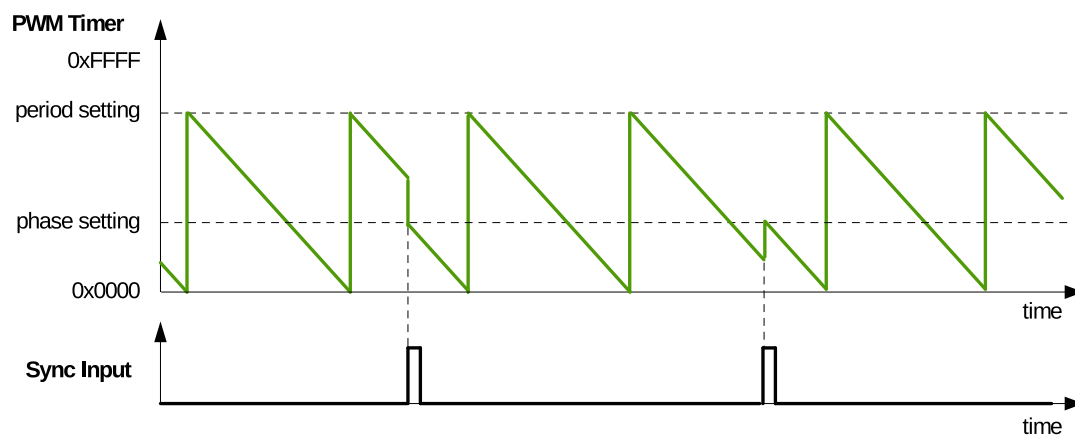
图 36.3-7. 递减计数模式波形
