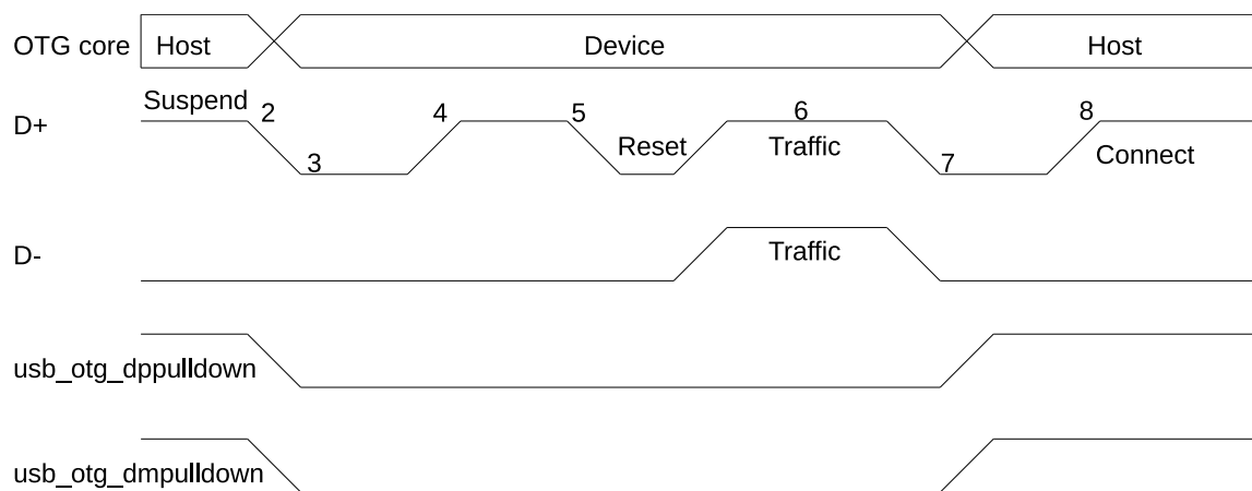
图 32.4-3. A 设备 HNP
