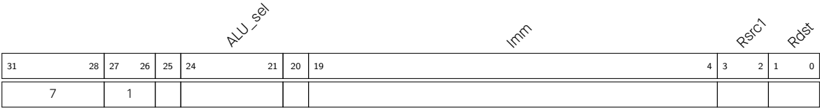
图 2.5-3. 指令类型 - 对指令立即值的 ALU 运算
