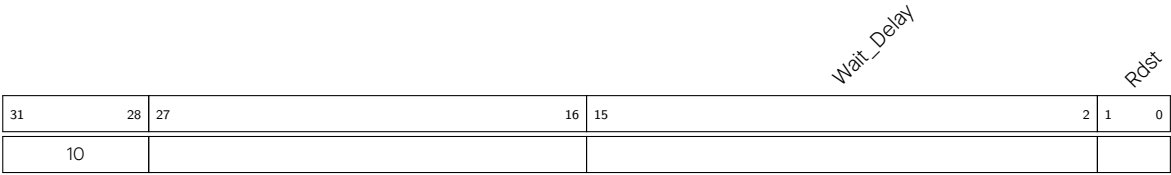
图 2.5-17. 指令类型 - TSENS
