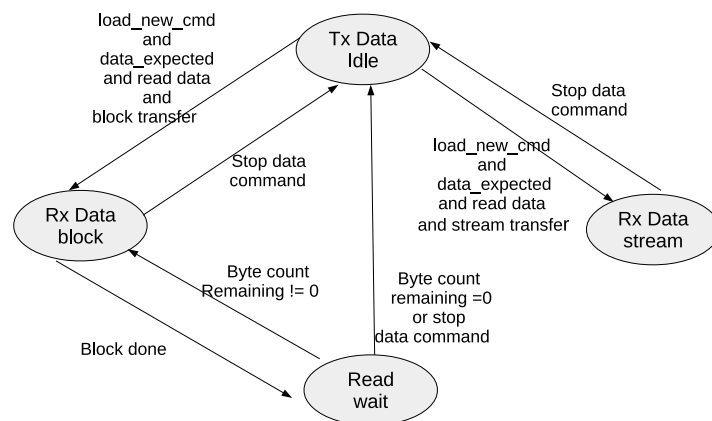
图 34.4-4. 数据接收状态机
