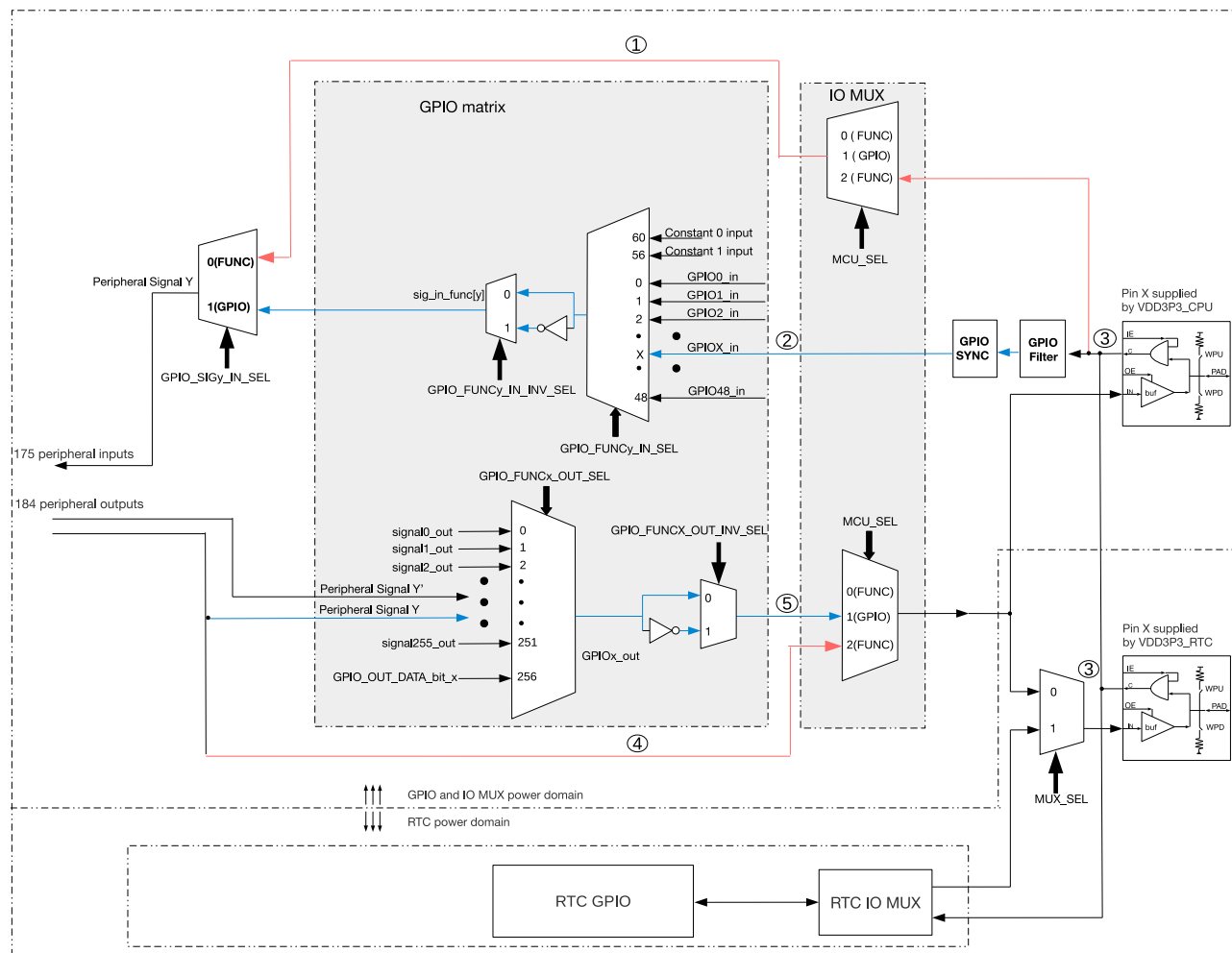
图 6.3-1. IO MUX、RTC IO MUX 和 GPIO 交换矩阵结构框图
