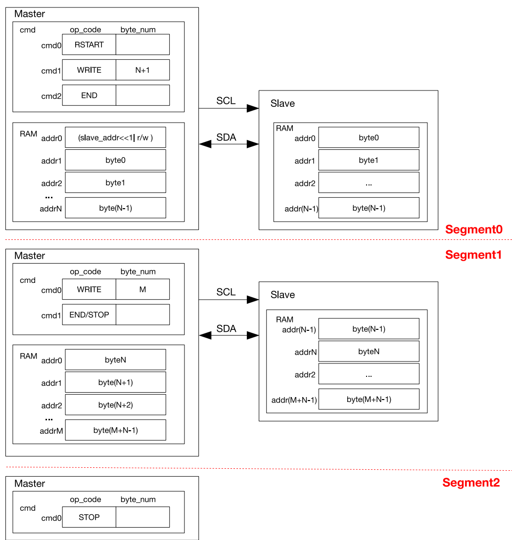
图 27.5-4. I2C 主机分段写 7 位寻址的从机
