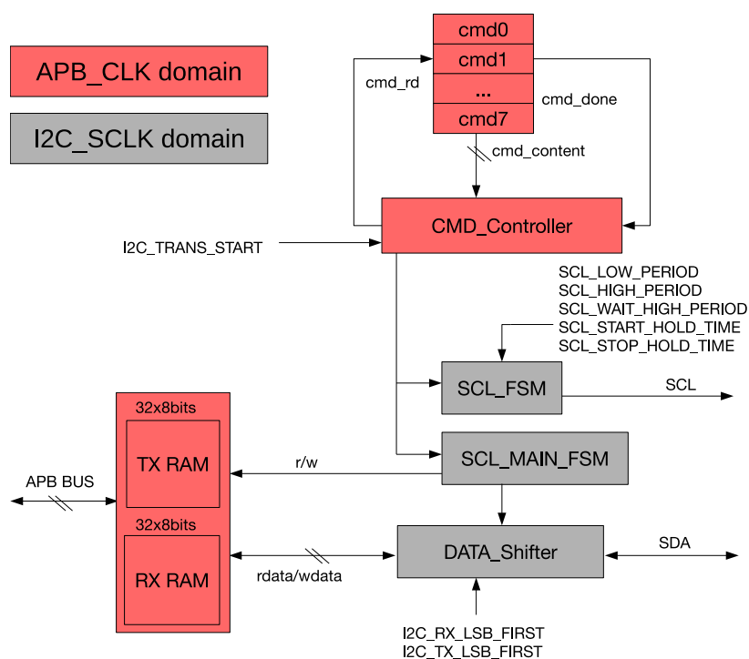
图 27.3-1. I2C 主机基本架构
