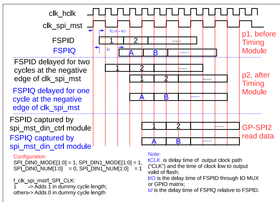
图 30.8-2. GP-SPI2 主机模式下时序补偿
