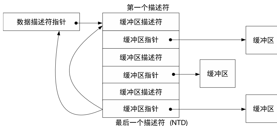
图 32.3-6. Scatter/Gather DMA 链表结构
