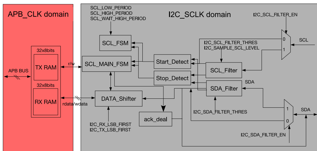
图 27.3-2. I2C 从机基本架构
