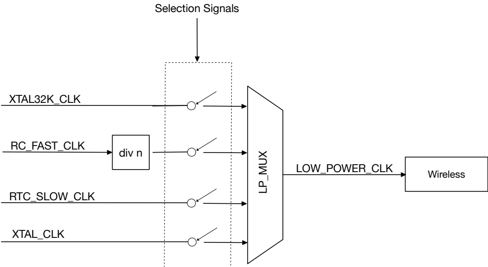
图 10.3-4. Wireless 时钟
