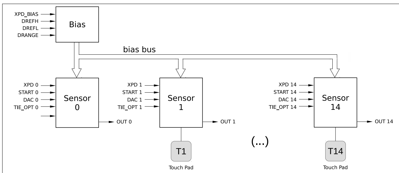
图 39.2-3. 触摸传感器的内部结构
