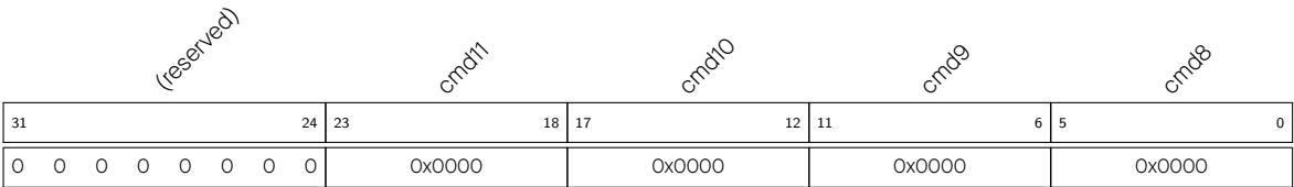
图 39.3-6. APB_SARADC_SAR1_PATT_TAB3_REG 与样式 8 - 11
