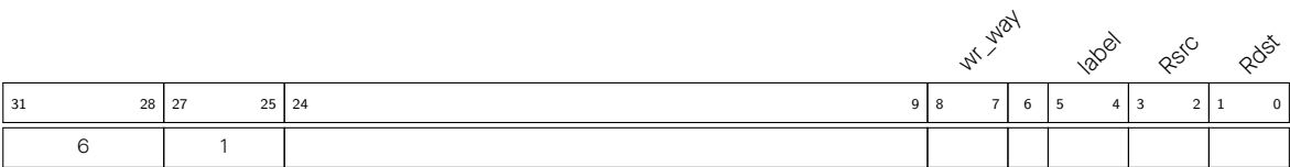
图 2.5-7. 指令类型 - 地址自增模式的数据存储 (ST-AUTO-DATA)
