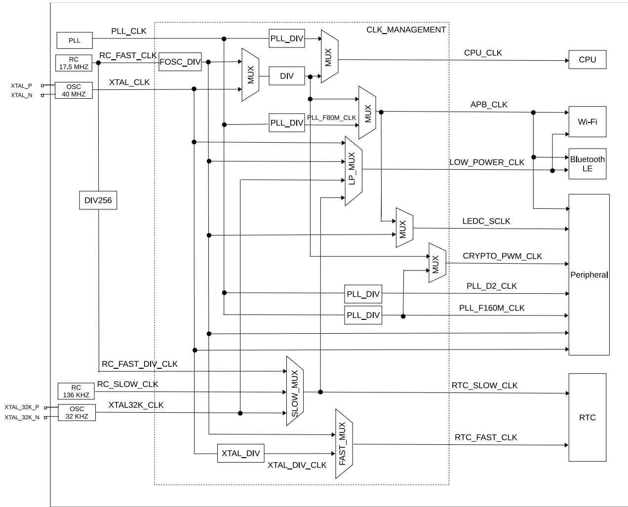
图 7.2-1. 系统时钟
