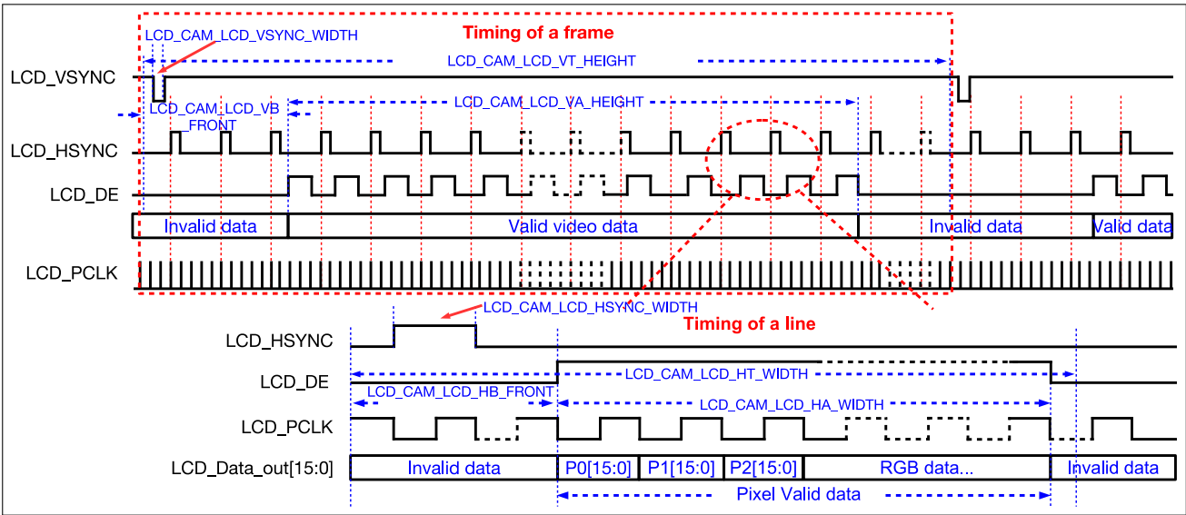
图 29.4-2. LCD 时序 (RGB 格式)
