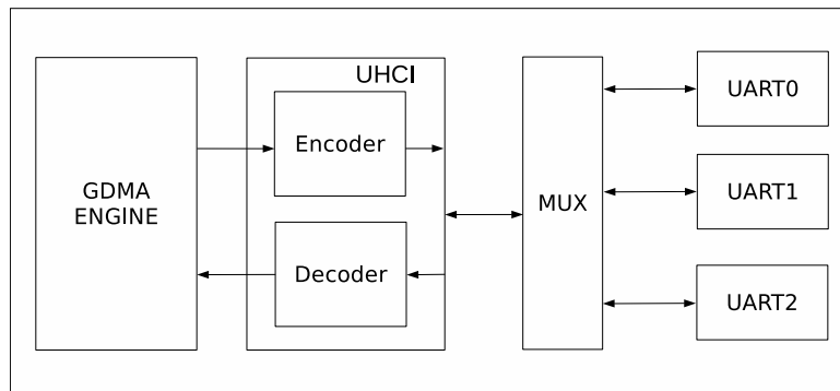
图 26.4-11. GDMA 模式数据传输
