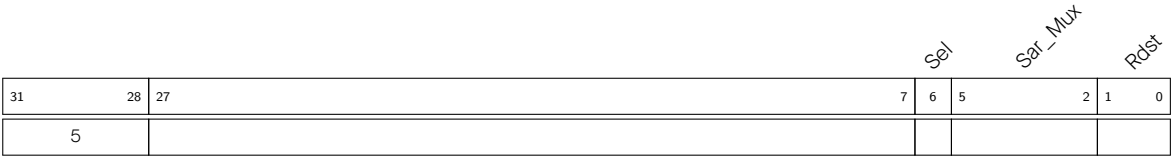
图 2.5-18. 指令类型 - ADC
