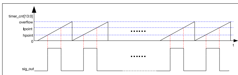
图 35.2-3. LED PWM 输出信号图
