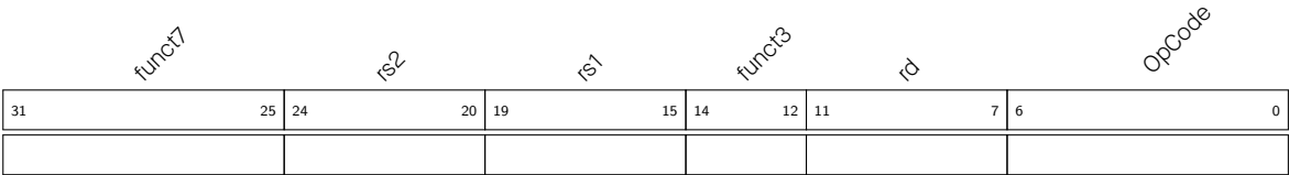
图 2.6-1. 标准 R-type 指令格式
