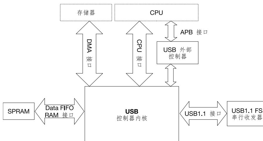
图 32.3-1. OTG_FS 系统架构
