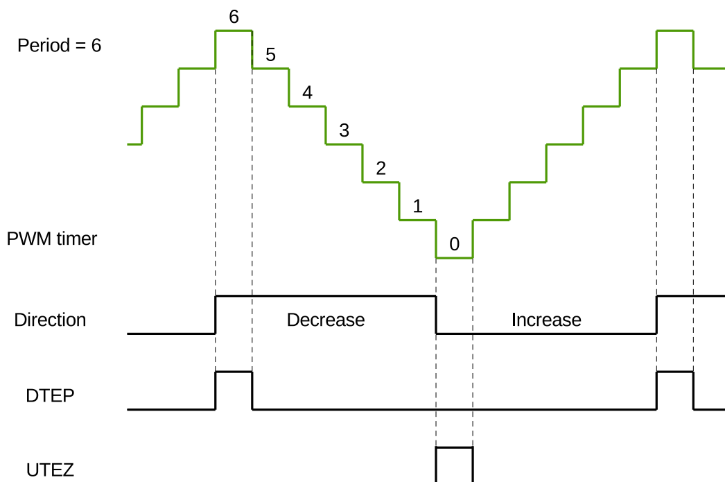
图 36.3-12. 递增递减模式中生成的 DTEP 和 UTEZ
