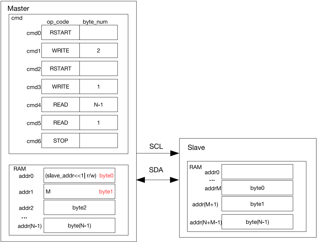
图 27.5-7. I2C 主机从 7 位寻址从机的 M 地址读取 N 个数据
