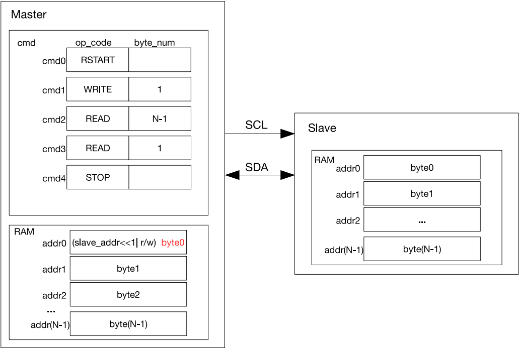
图 27.5-5. I2C 主机读 7 位寻址的从机
