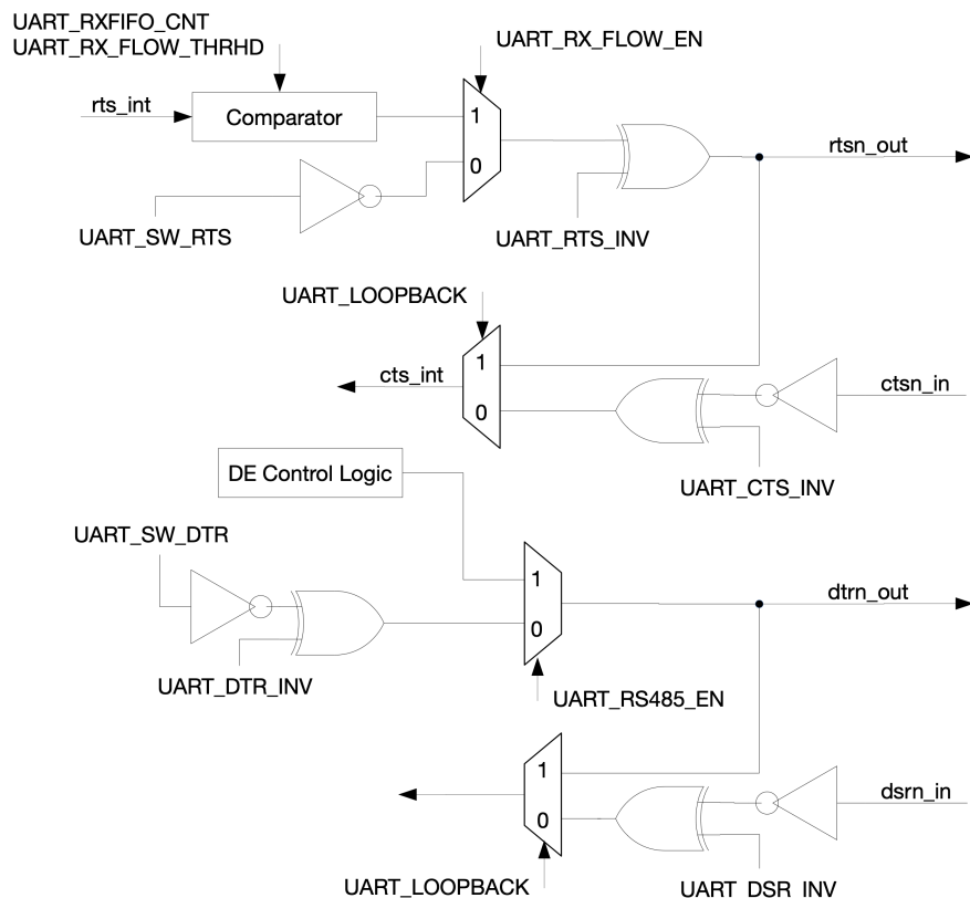
图 26.4-9. 硬件流控图
