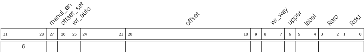
图 2.5-5. 指令类型 - ST
