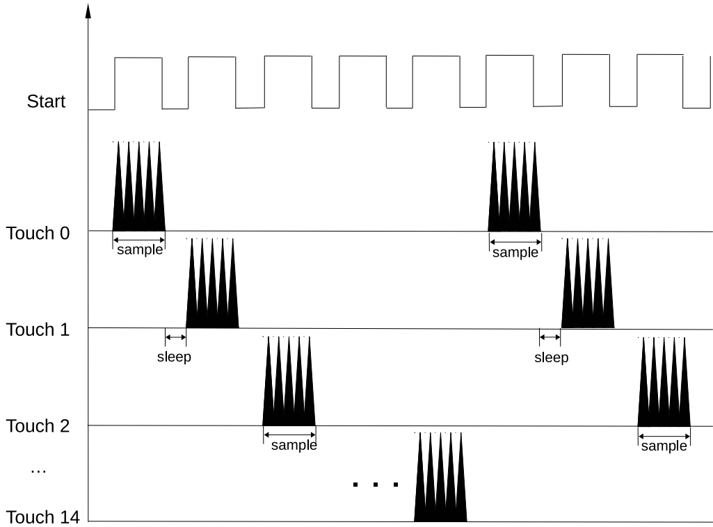
图 39.2-5. TOUCH SCAN 时序图
