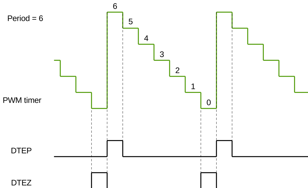
图 36.3-11. 递减模式中生成的 DTEP 和 DTEZ
