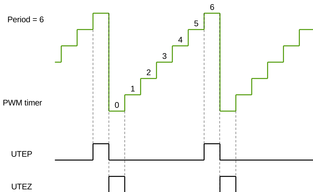
图 36.3-10. 递增模式中生成的 UTEP 和 UTEZ
