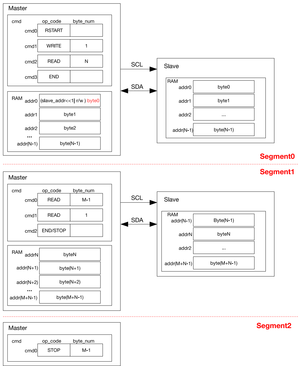
图 27.5-8. I2C 主机分段读 7 位寻址的从机
