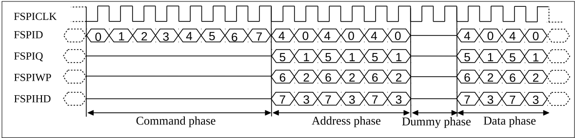
图 30.5-8. GP-SPI2 发送到 flash 的 SPI Quad I/O Read 命令序列
