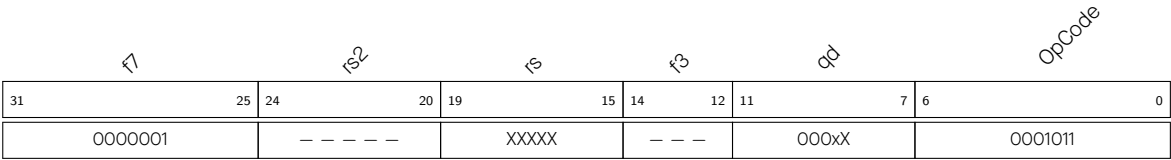
图 2.6-3. 中断指令 - setq qd, rs
