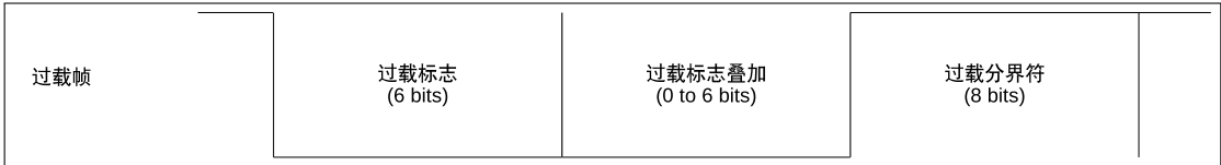
图 31.3-3. 过载帧中的位域
