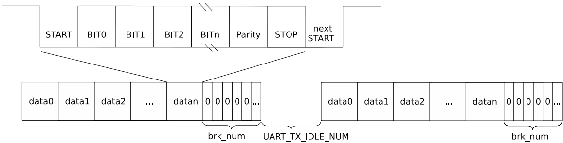
图 26.4-4. UART 数据帧结构
