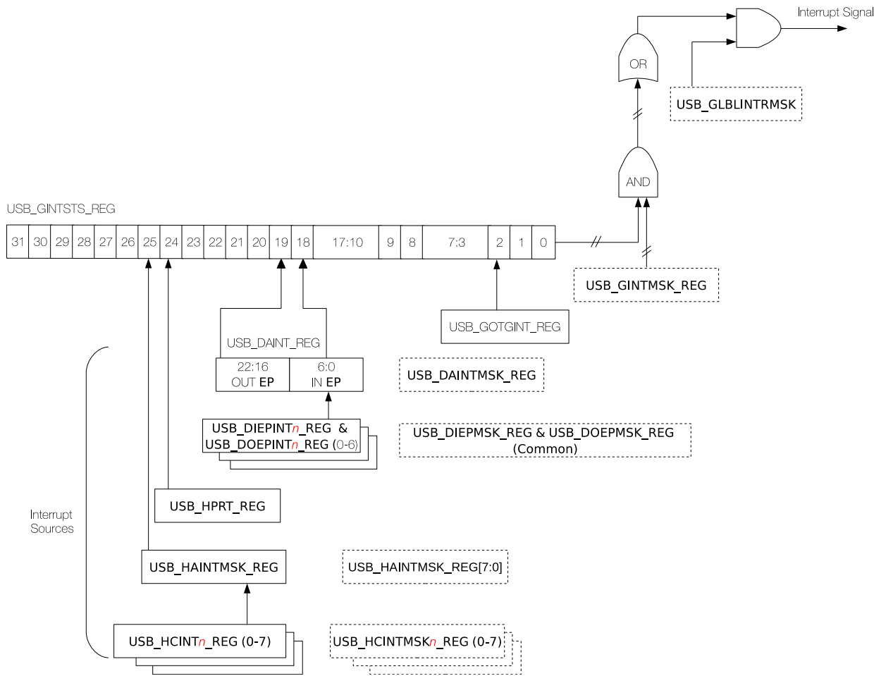
图 32.3-5. OTG_FS 中断层次结构图
