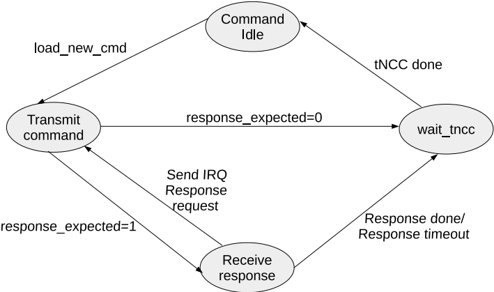
图 34.4-2. 命令通路状态机
