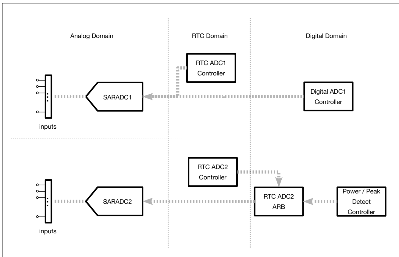
图 39.3-1. SAR ADC 概图
