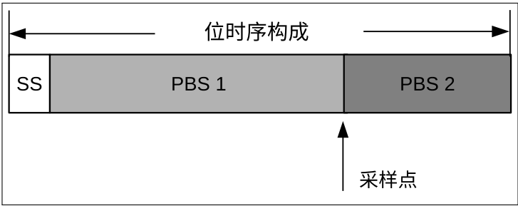
图 31.3-5. 位时序构成
