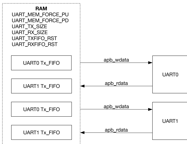
图 26.3-1. UART 架构概况
