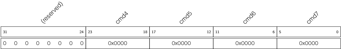
图 39.3-5. APB_SARADC_SAR1_PATT_TAB2_REG 与样式 4 - 7
