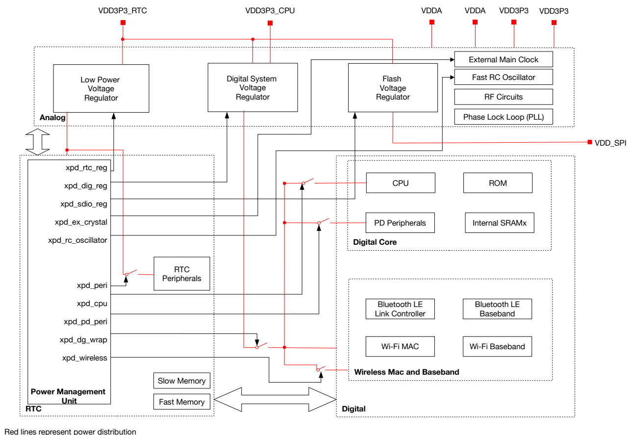
图 10.3-1. 低功耗管理原理图
