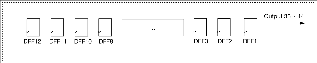
图 5.3-2. 移位寄存器电路图（后 12 字节）
