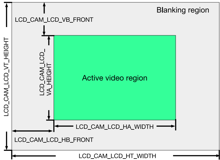
图 29.4-1. LCD 视频帧结构
