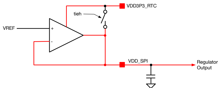
图 10.3-7. flash 调压器
