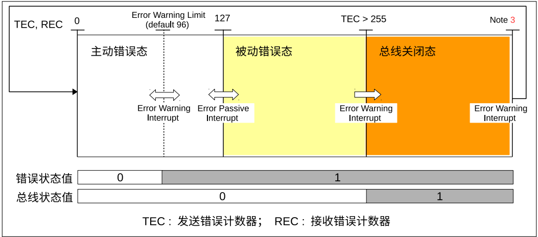
图 31.5-4. 错误状态变化
