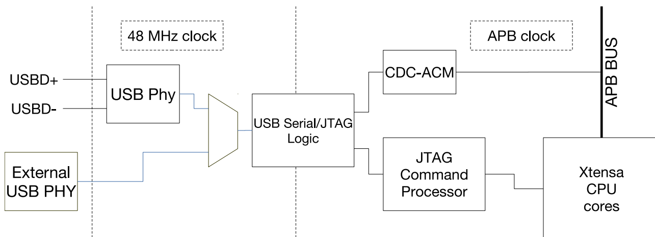
图 33.2-1. USB Serial/JTAG 高层框图
