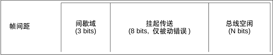
图 31.3-4. 帧间距中的域
