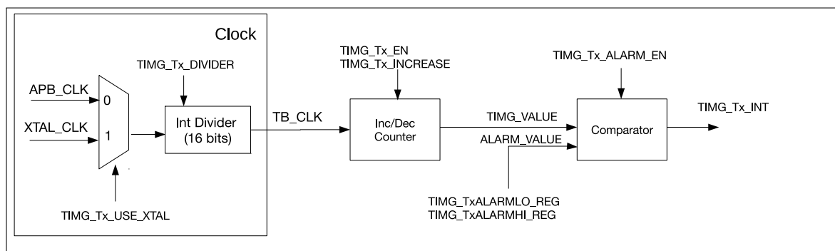
图 12.2-1. 定时器组架构
