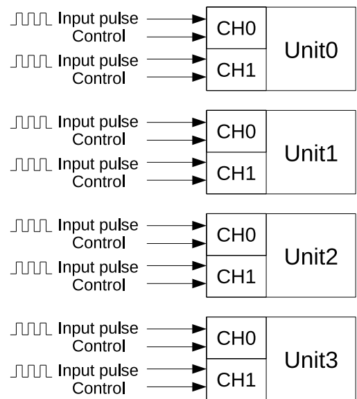
图 38.0-1. PCNT 框图
