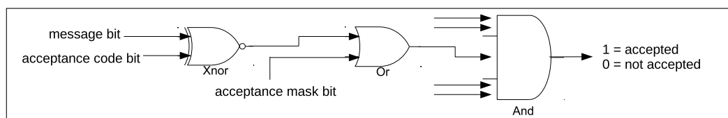
图 31.5-1. 接收滤波器
