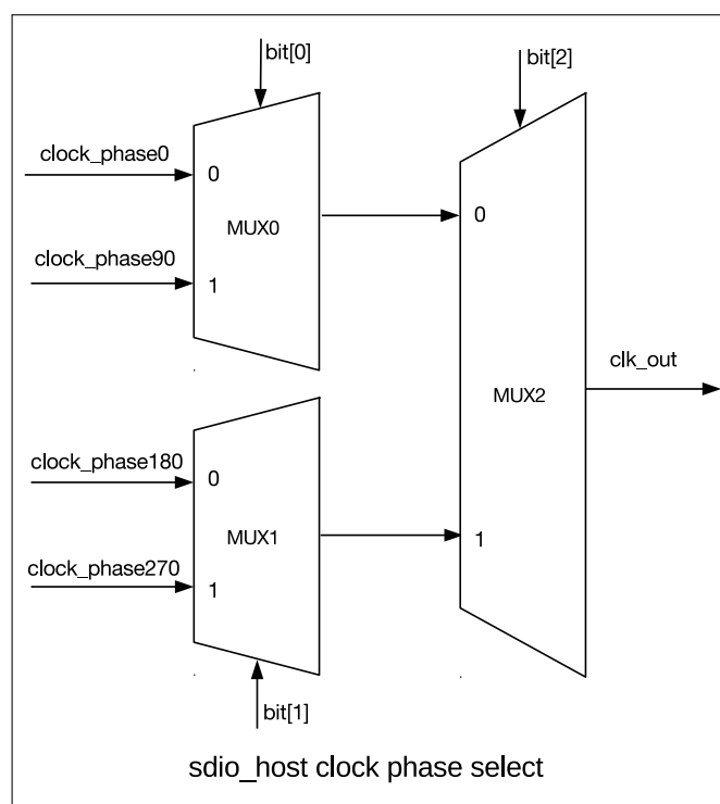
图 34.10-1. 时钟相位选择
