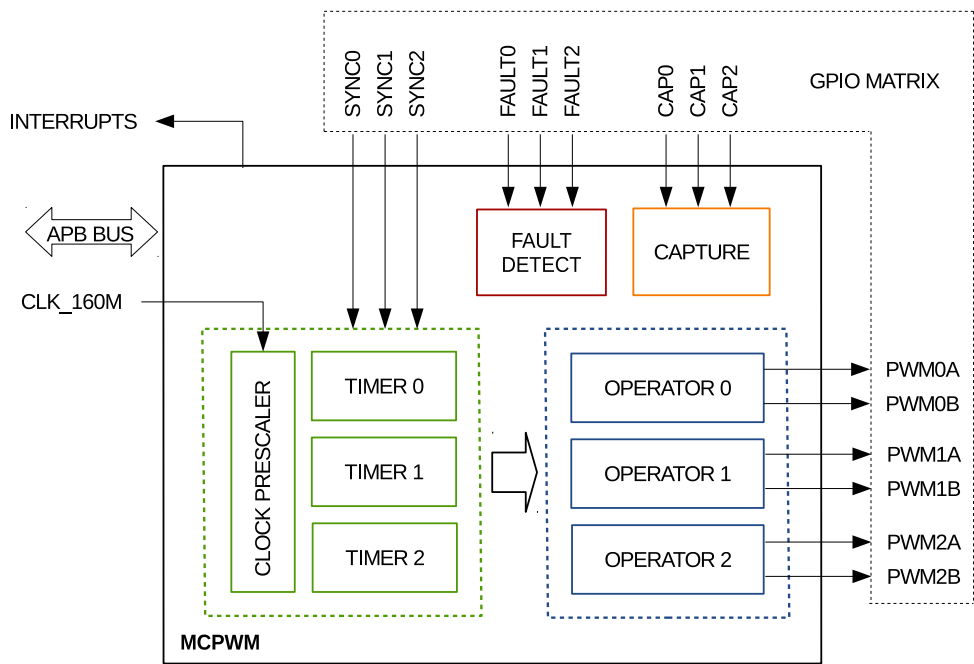
图 36.2-1. MCPWM 外设概览
