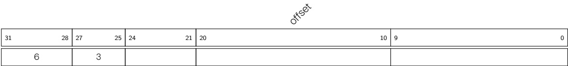
图 2.5-6. 指令类型 - 地址自增模式的基地址偏移 (ST-OFFSET)
