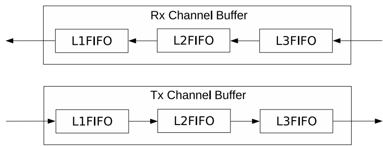
图 3.4-2. 通道 Buffer 示意图
