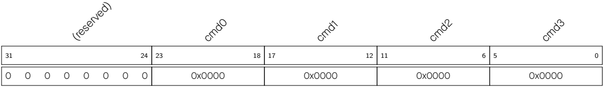
图 39.3-4. APB_SARADC_SAR1_PATT_TAB1_REG 与样式 0 - 3
