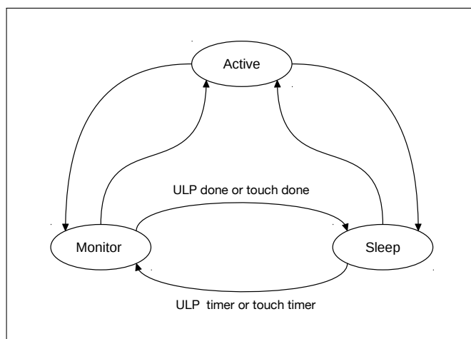
图 10.4-1. RTC 状态
