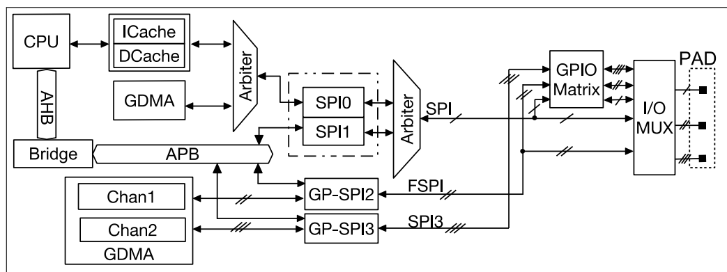
图 30.4-1. SPI 模块概览
