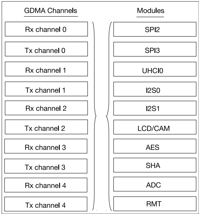
图 3.1-1. 具有 GDMA 功能的模块和 GDMA 通道
