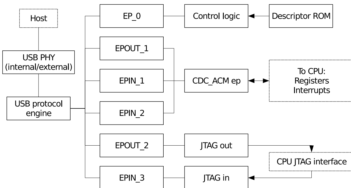
图 33.2-2. USB Serial/JTAG 框图
