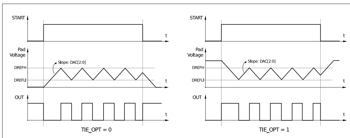
图 39.2-2. 触摸传感器工作原理
