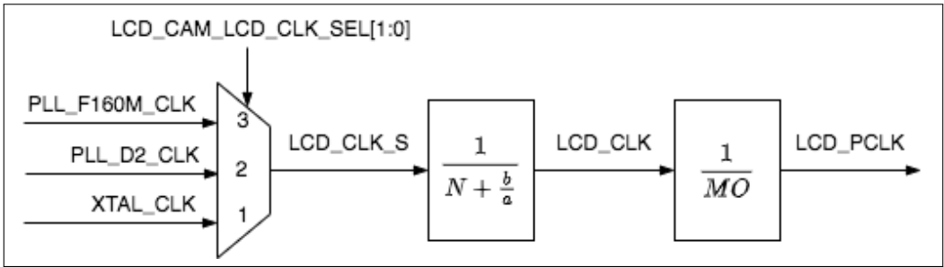
图 29.3-2. LCD 时钟
