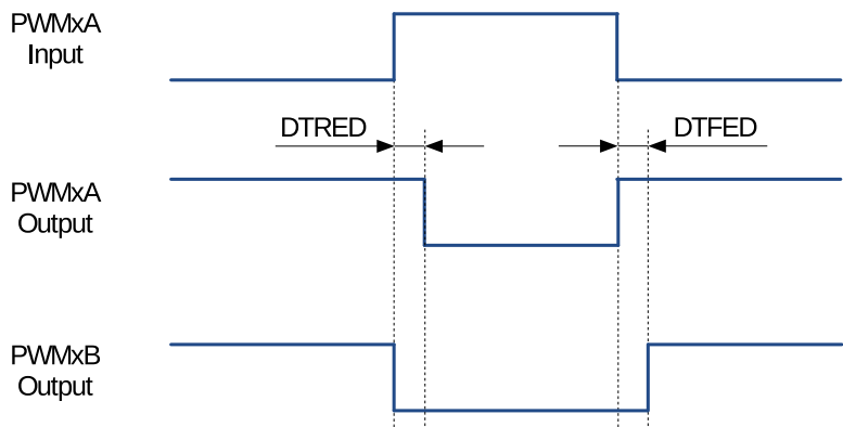
图 36.3-25. 低电平有效 (AL) 死区波形
