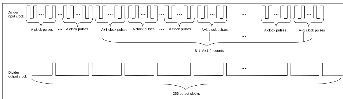
图 35.2-2. LEDC_CLK_DIV 非整数时的分频
