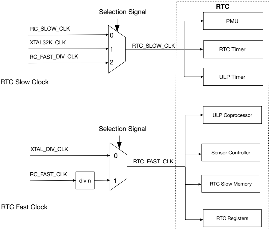
图 10.3-3. RTC 时钟
