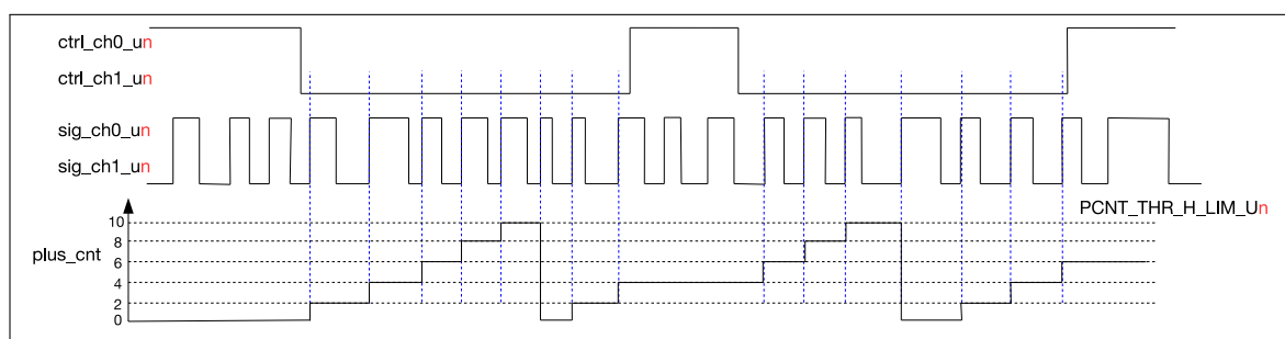
图 38.3-3. 双通道递增计数图
