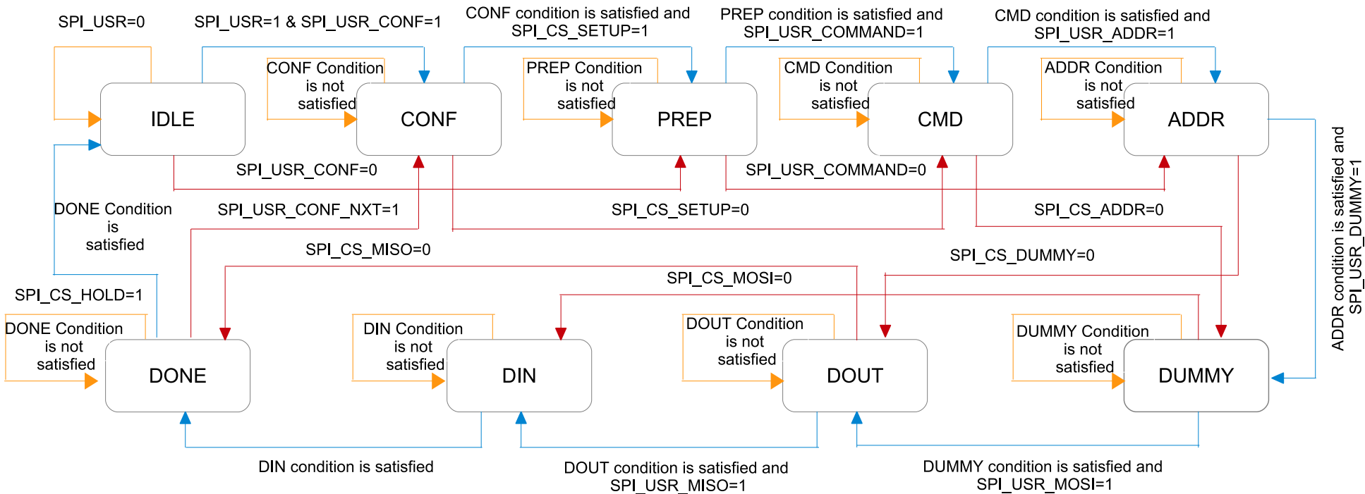
图 30.5-5. GP-SPI 主机模式状态机
