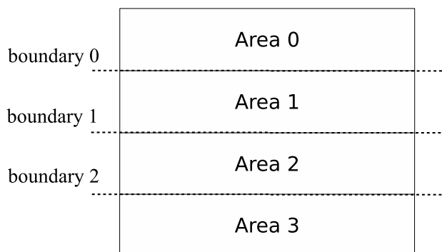
图 3.4-4. 外部 RAM 的权限区域划分
