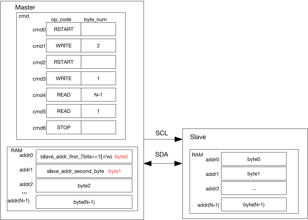
图 27.5-6. I2C 主机读 10 位寻址的从机
