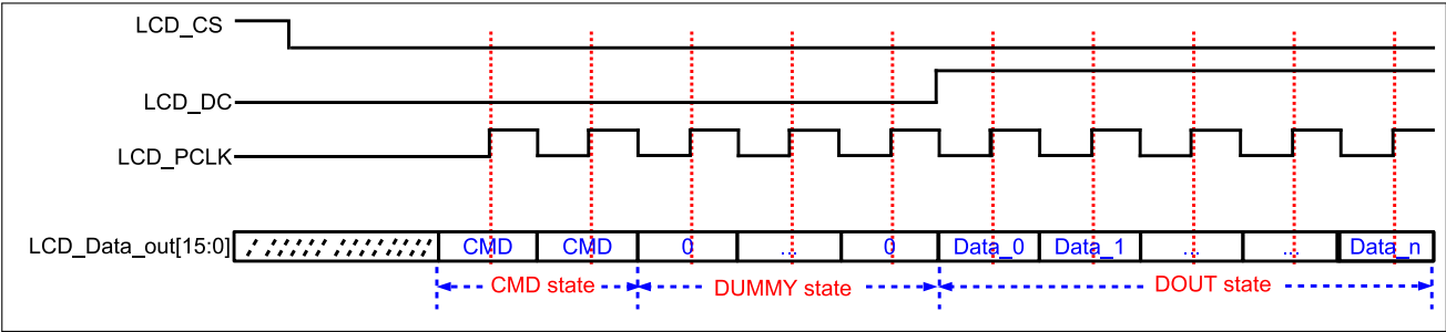
图 29.4-3. LCD 时序 (I8080 格式)
