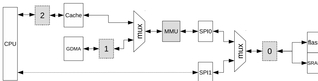
图 15.5-1. 外部存储器访问路径示意图
