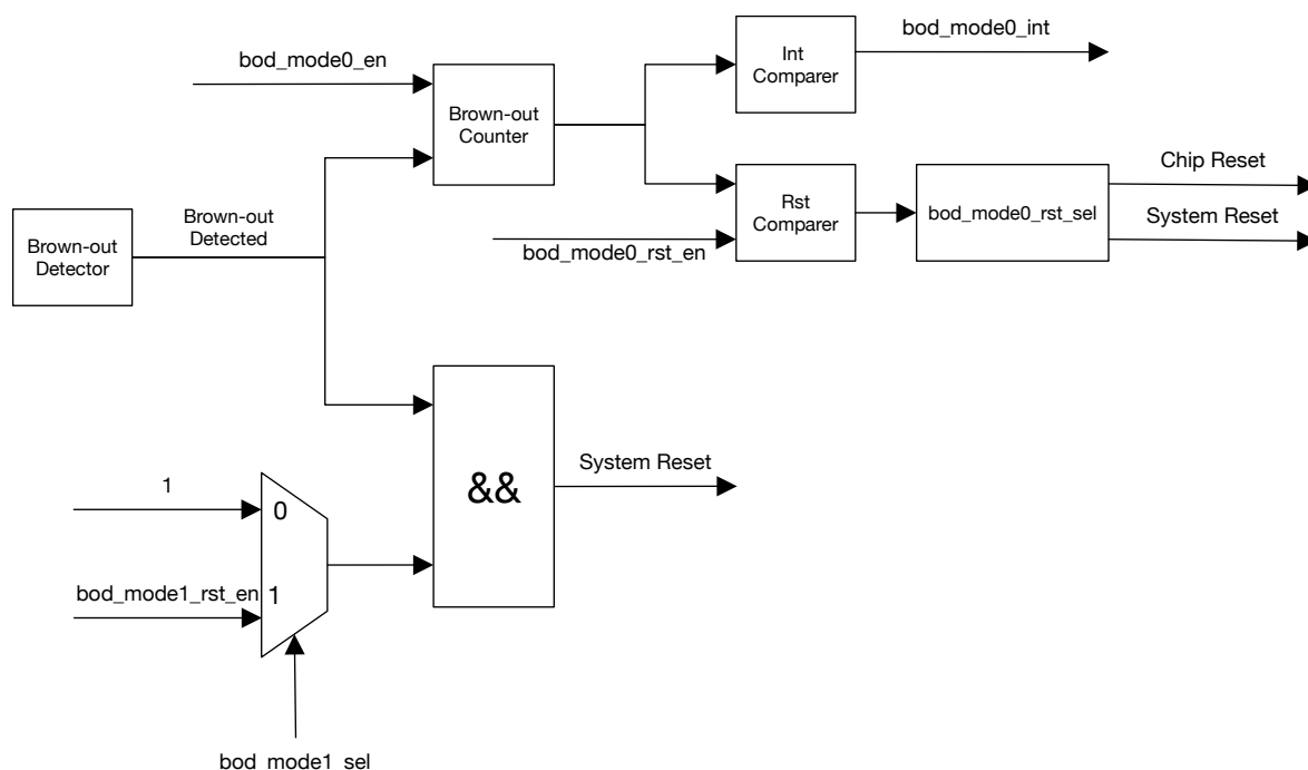
图 10.3-9. 欠压检测器处理方式
