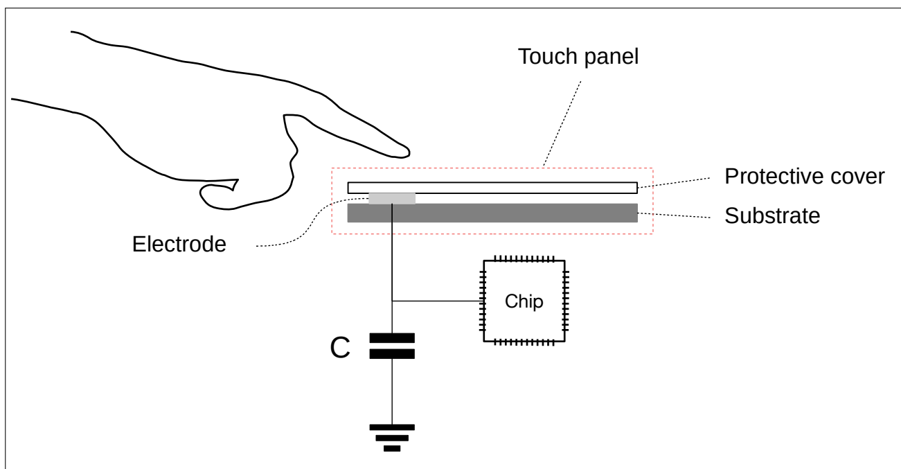
图 39.2-1. 触摸传感器
