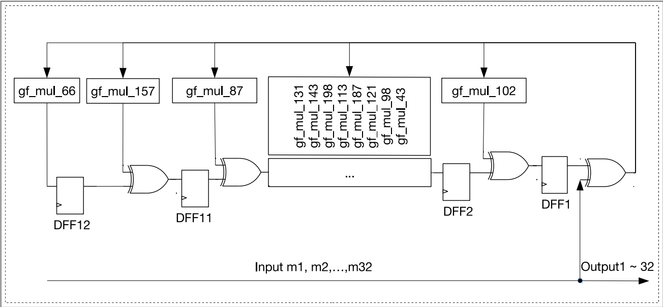
图 5.3-1. 移位寄存器电路图（前 32 字节）
